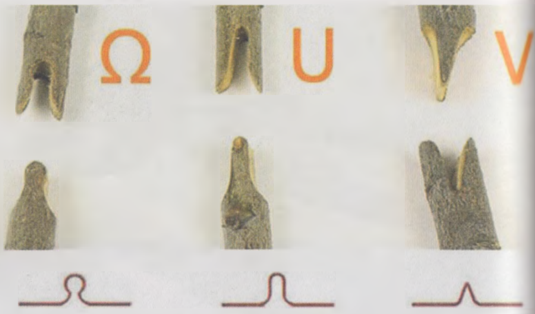
18-расм. Махсус пайвандлаш қайчи билан новдани фигурали кесилиши ва пайвандлаш
