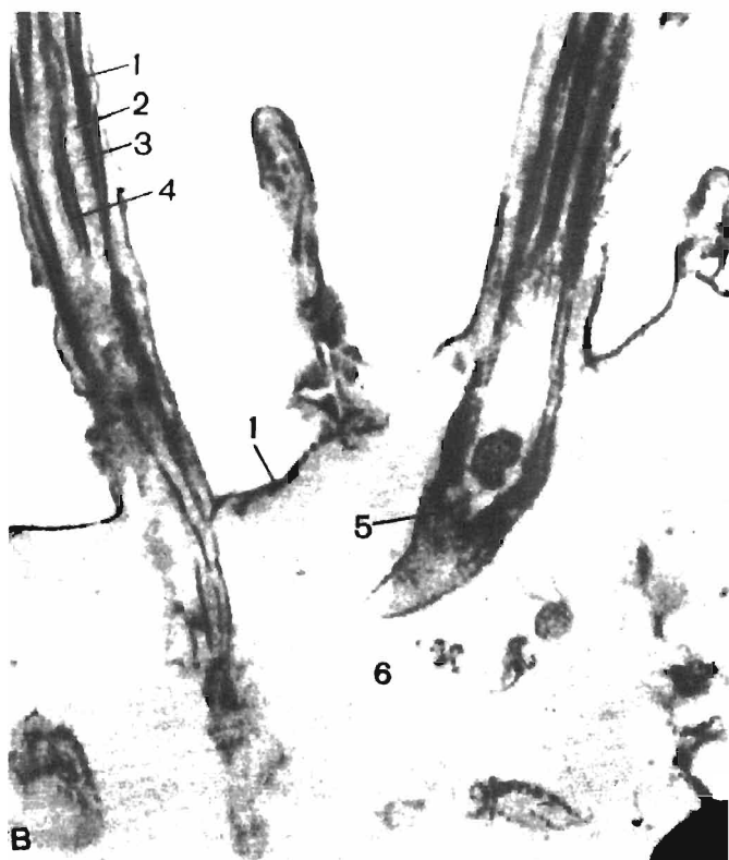
91-rasm. Hujayra kipriklari. A-kiprikchanning ko'ndalang kesimi x96000; b-kiprikchanning uzunasiga kesimi — x68000. 1-sitolemma; 2-kiprik sitoplazmasi; 3-mikrofibrillar; 4-markaziy mikro fibril; 5-bazal tanacha; 6-hujayraning distal bo'limi
