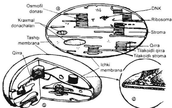
17a-rasm. Xloroplastning tuzilishi.
