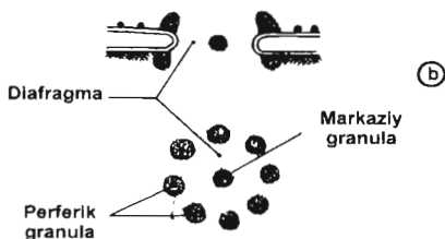
36-rasm. Yadro membranasi poralari (teshikchalari) chizmasi. a-halqali zich moddali ochiq pora; b-diafragmalı pora
