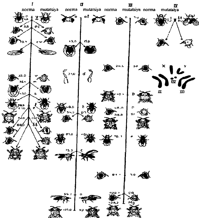
34 - rasm. Drosophila xromosomasining genetik xaritasi. Raqamlar genlar orasidagi masofani va xromosomadagi oxirgi raqam ularning chalkashuv birlikini ifodalaydi.
