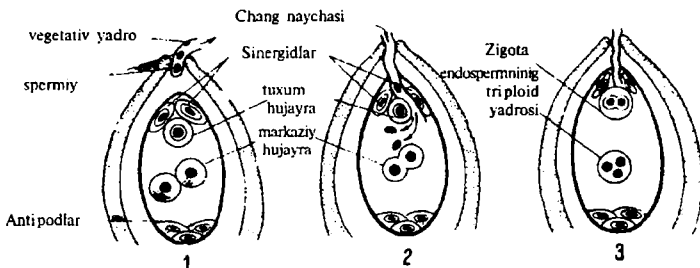
12 - rasm. O'simliklarning qo'sh urug'lanish sxemasi. 1 — chang naychasing murtak xaltachasiga o'sib kirishi. 2 — naycha ichidagi spermialarning murtak xaltachasiga quyilishi. 3 — urug'lanishdan so'ng murtak xaltachasi.
