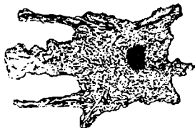
51-rasm. Somatik mutatsiya (Qorako'l qo'ylar yungida qora dog'lar bo'lishi).
