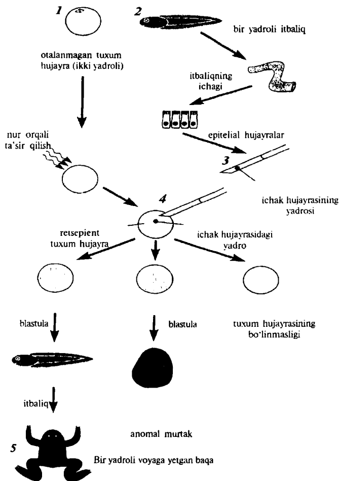
65 - rasm. Itbaliqning ichagidan olingan yadroni baqaning o'talmagan tuxum hujayrasiga ko'chirish sxemasi. Dj. Gerdon tajribasi.
