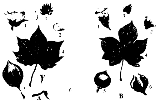
54 - rasm. G'o'zaning tetraploid (A) va diploid (B) turlari: G.hirsutum L. va G.herbaceum L. 1 - guli, 2 - gultojibargi, 3 - gulqo'rg'oni, 4 - bargi, 5 - ochilmagan ko'sagi, 6 - ochilgan ko'sak.
