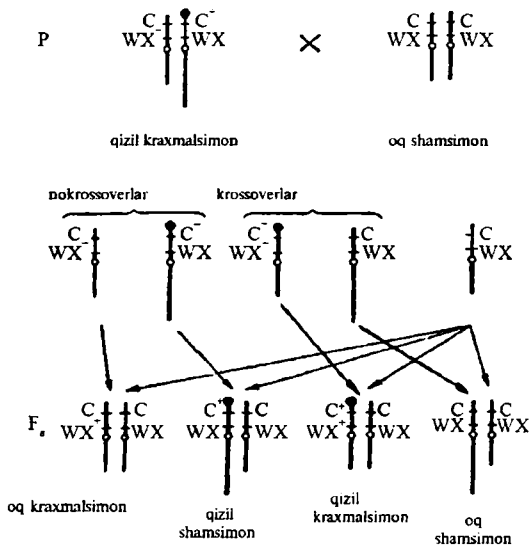
32 - rasm. Makkajo 'xorida crossingoverning sitologik isboti. C^+ - endospermi qizil, C - endospermi oq, WX^+ - endospermi kraxmalsimon, WX - endospermi shamsimon.
