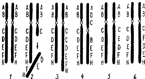
52 - rasm. Xromosomalarning qayta tiklanishi. 1 – dastlabki gomologik xromosomalarning jufti. 2 – DEFH qismining uzilishi. 3 – C qismining duplikatsiyasi. 4 – BCD qismining inversiyasi. 5 – DE qismining inversiyasi. 6 – inversiya DE qismining qayta joylashishi.
