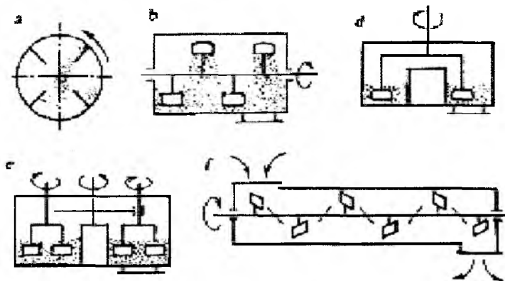
4.45-rasm. Aralashmani qo'zg'atish usullarining prinsiplial chizmalari: a—gravitatsion beton qorgichlar; b, d—parraklarga ega bo'lgan gorizontal valli; e, f—parraklarga ega bo'lgan rotorli.
