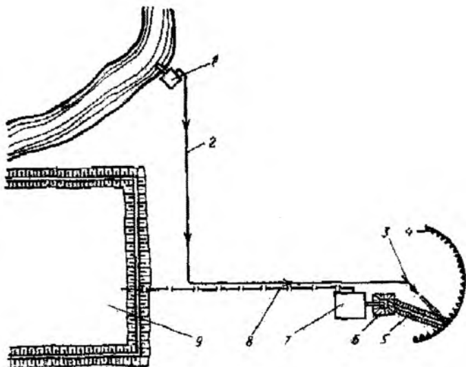
4.38-rasm. Hidromonitor usulida gruntni ishlash sxemasi.
