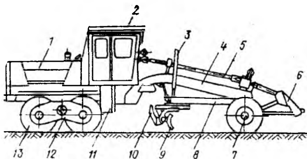
4.18-rasm. DZ-99-1-4 avtogreyderi:
