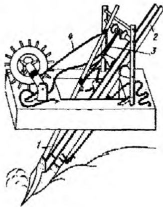
3.14-rasm. D.Fontanning suzuvchi bir cho'michli ekskavatorining prototipi (1420-y.): 1—tyaga; 2—tirsak; 3—ish jihazini tortuvchi arqon; 4—napor hosil qiluvchi arqon.
