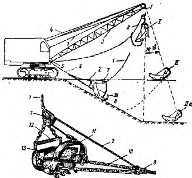
4.26-rasm. Draglaynli bir kovshli ekskavatorning konstruktiv sxemasi: I—osilgan kovshning vaziyati; II—kovsh qazimaga tushirilgan, III—gruntni olish; 1, 2, b—ko'taruvchi, bo'shatuvchi va tortuvchi kanatlar; 3—strela, 4—strela osiladigan kanatlar; 5—yo'naltiruvchi qurilma, 7—kovshni ko'taruvchi blok; 8—kovsh; 9—zanjirni kovshga mahkamlagich; 10, 13—tortuvchi va ko'taruvchi zanjirlar; 11—arka; 12—traversalar.
