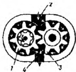
4.27-rasm. Shesternyali nasos sxemasi:
