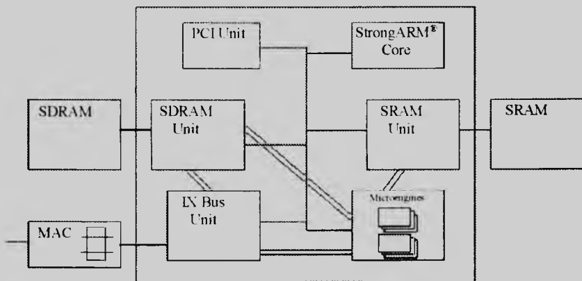
3.9-chizma. IXP1200 protsessorida paketga ishlov berish
