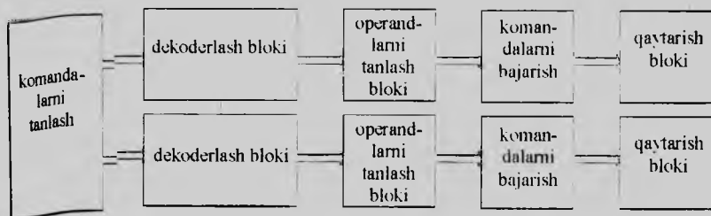
1.10.-chizmi. Komandalarni chaqiruvchi umumiy bo'limga ega besh bosqichdan iborat ikkitalik konveyer
