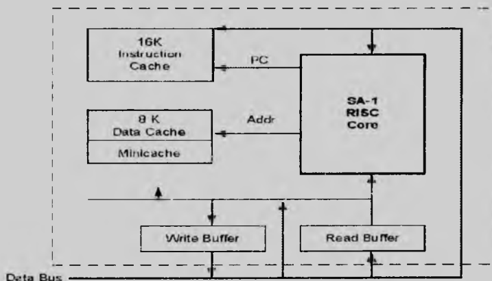
3.4-chizma. StrongARM mikroprotessori blok-sxemasi
