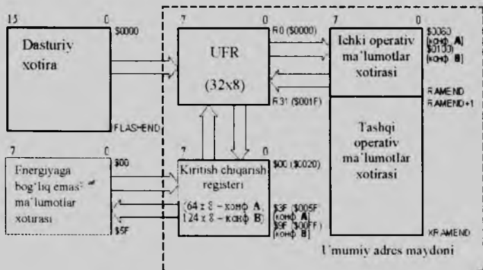
4.13-chizma. AVR-mikrokontrollerlarning dasturiy modeli
