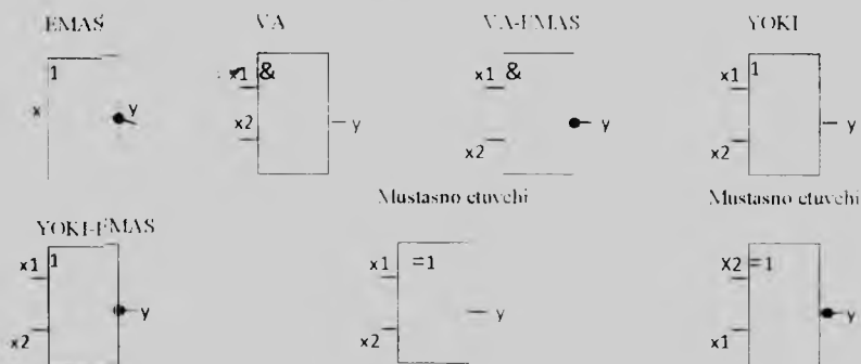
1.2-chizma. Mantiqiy elementlarning shartli belgilanishlari
