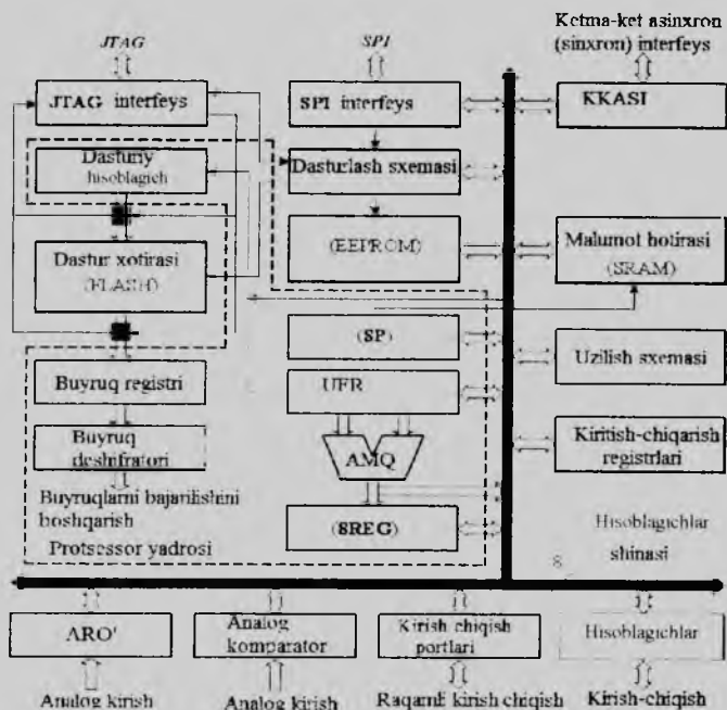
4.12-chizma. AVR oilasiga mansub mikrokontrollerlarning strukturasi
