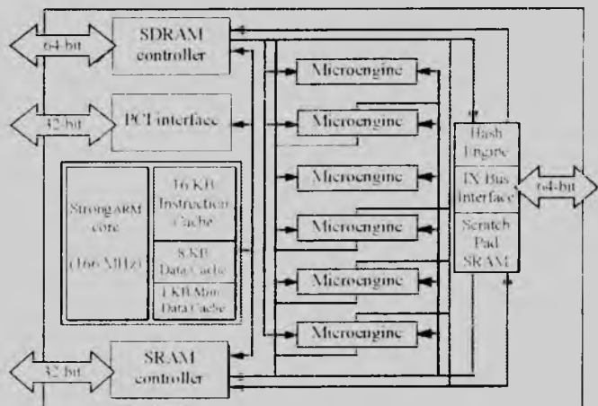
3.5-chizma. IXP1200 mikroprotessori blok-sxemasi
