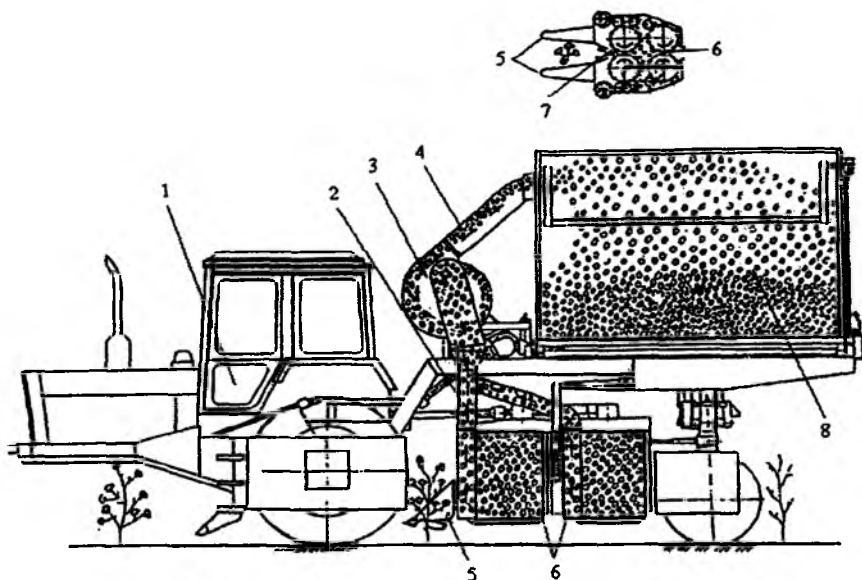
2.30-rasm. MX-1,8 rusumli paxta terish mashinasi (a) va terish apparatining (b) texnologik sxemasi: 1 – traktor; 2 – soʻruvchi kanal; 3 – ventilyator; 4 – haydovchi kanal; 5 – gʻoʻzapoya koʻtargich; 6 – vertikal shpindelli terish apparati; 7 – tik shpindelli barabanlar; 8 – bunker.
