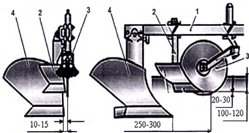
2.3-rasm. Plugning asosiy qismlari va ularni roslash o'lchamlari: 1 – rama; 2 – chimqirqar; 3 – diskli pichoq; 4 – asosiy korpus.
