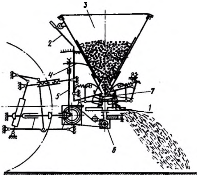
2.14-rasm. NRU-0,5 diskli o'g'it sochgich sxemasi:
