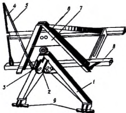
1.17-rasm. Traktor avtosepkasi:
