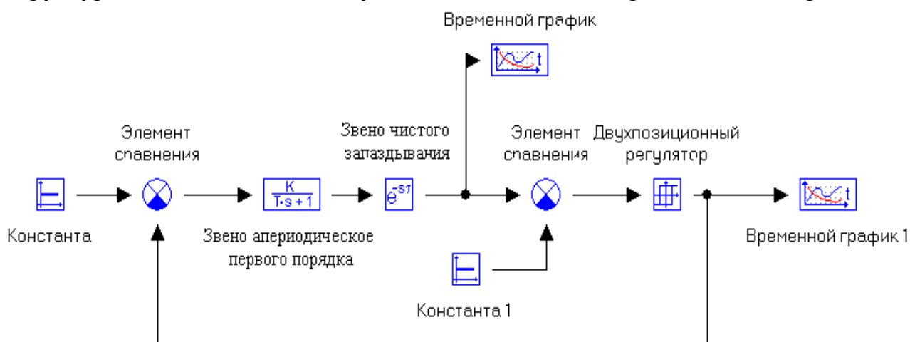
Рисунок 1. – Структурная схема модели обычной двухпозиционной САР.
