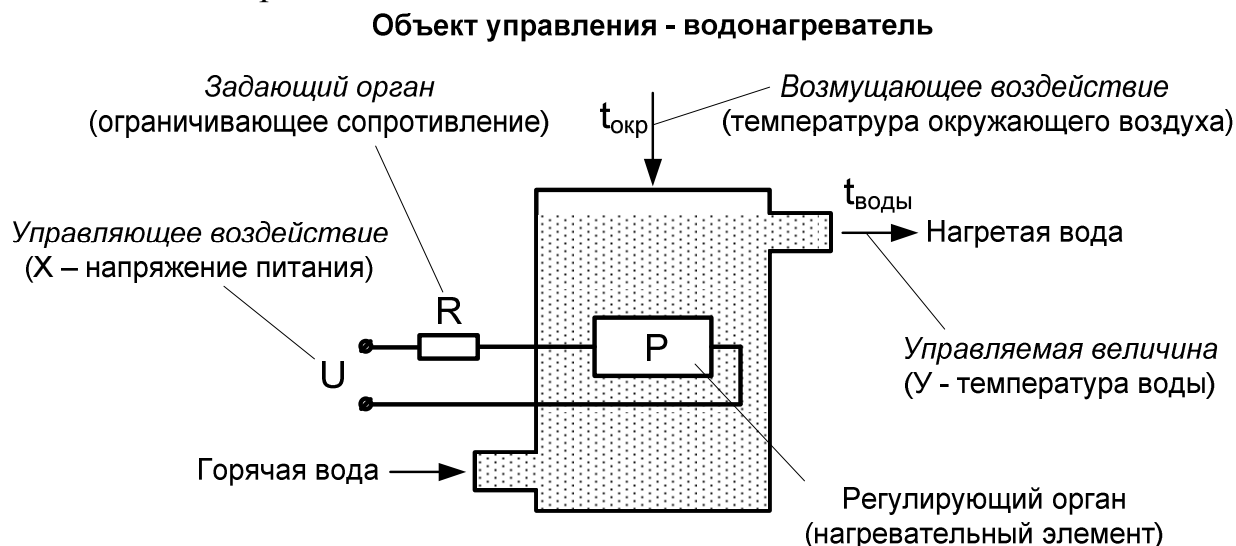
Рисунок 1 - Водонагреватель как объект управления (P - мощность нагревательного элемента)
