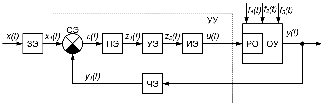
Рисунок 7 - Замкнутая САУ
