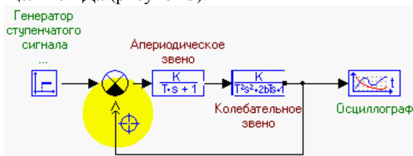
Рисунок 2 – Порядок создания ветвления и проведения линии связи.
