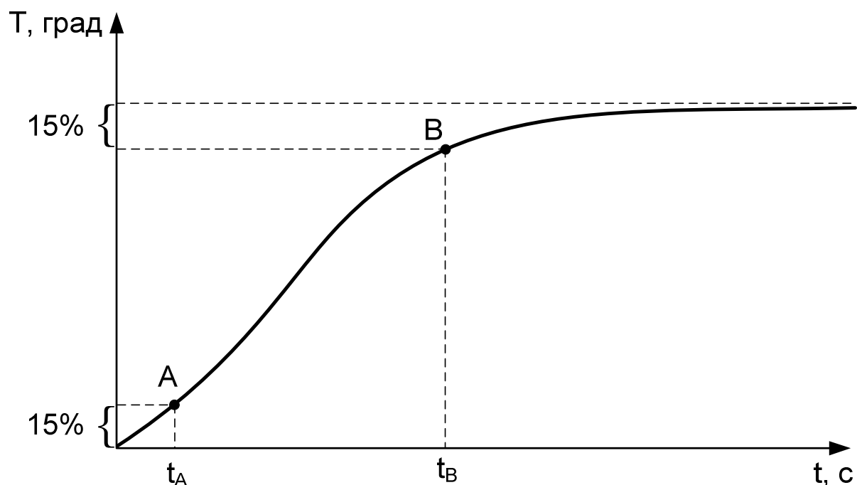
Рисунок 11 – Нахождение T_{OУ} и \tau .
