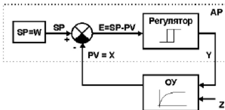
Рисунок 3 - Структурная схема двухпозиционной системы регулирования. где: AP – двухпозиционный регулятор, ОУ – объект управления, SP – уставка, E – рассогласование регулятора, PV=X – контролируемая величина, Y – управляющее воздействие, Z – возмущающее воздействие.
