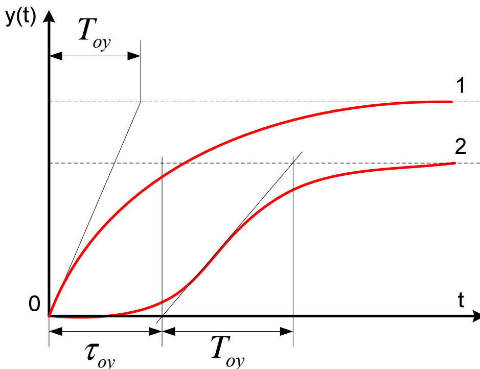
Рисунок 15 - Пример двух объектов с разными динамическими свойствами. ( T_{ou} - постоянная времени объекта управления \tau_{ou} - время чистого запаздывания объекта управления)
