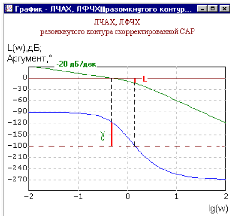
Рисунок 15 – ЛАЧХ и ЛФЧХ скорректированной САР.
