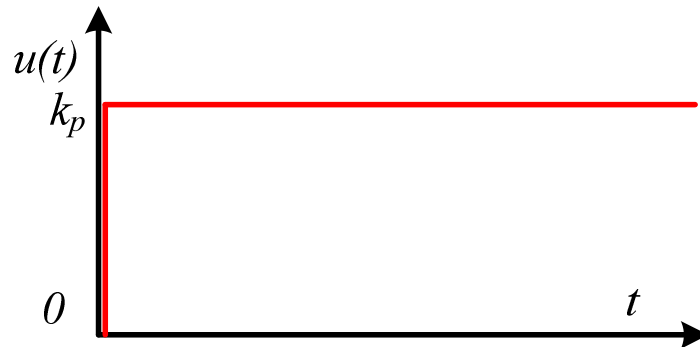
Рисунок 2 – Переходная характеристика П-регулятора.
