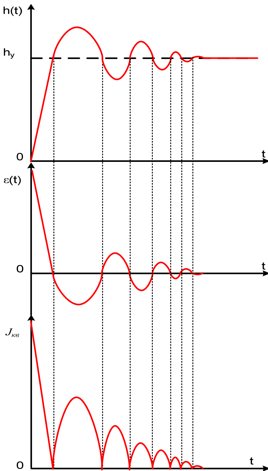
Рисунок 13 - Обобщенный интегральный среднеквадратичный показатель J_{кв}
