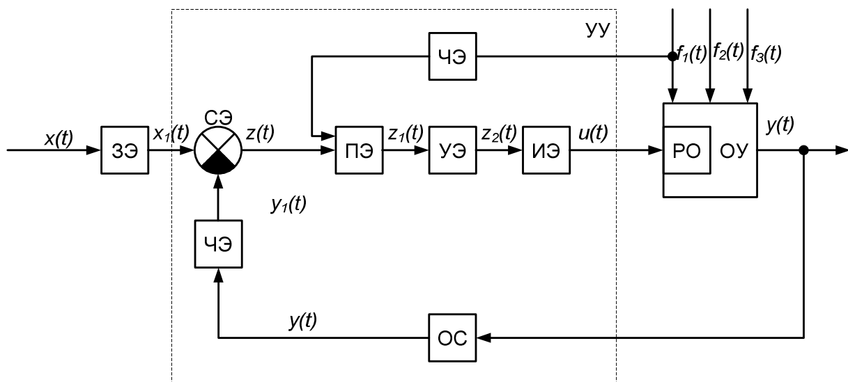
Рисунок 8 - Комбинированная САУ
