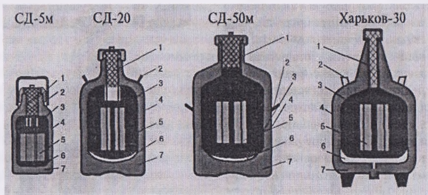
11-rasm. Spermani saqlash va tashishga muljallangan D'yuar sosudlarining turli konstruktsiyalari. 1-qopqoq; 2-ruchka; 3-4-ichki va tashqi sosudlar; 5-kanistr; 6- adsorbentli kamera; 7-issiqlik o'tkazmaydigan material.
