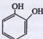
orto-dioksibenzol (pirokatexin)
