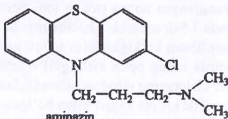
aminazin
