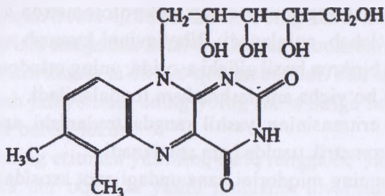
izoriboflavin
