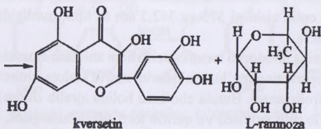
L-rannoza
