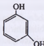
meta-dioksibenzol (rezorsin)
