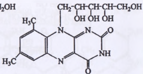
6,8-dimetil-9-pibitilizoalloksazin
