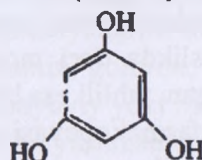
1,3,5-trioksibenzol (floraglutsin)
