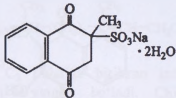
vikasol
