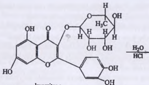
kversitron
