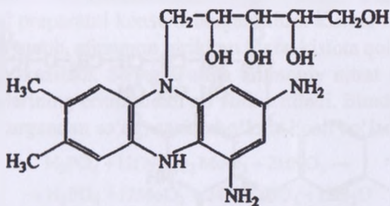
2,4-diamino-6,7-metil-9-ribitil-digidrofenazin
