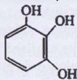
1,2,3-trioksibenzol (pirogallol)
