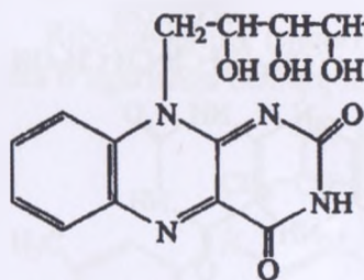
9-pibitilizoalloksazin
