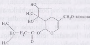
Валерозидат
