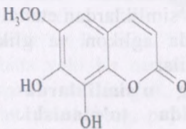
Фраксетол
