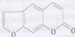
Псорален (фуранокумарин)
