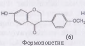
Формонететин
