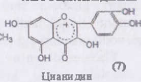
Цианидин
