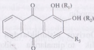
Ализарин
