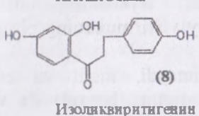
Изоликвиртетин
