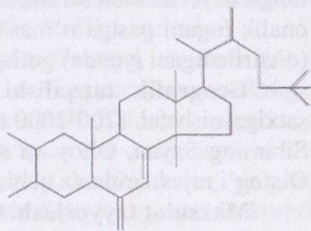
α-Экдиол
