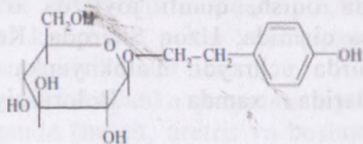
Салидрозид (розинолид)
