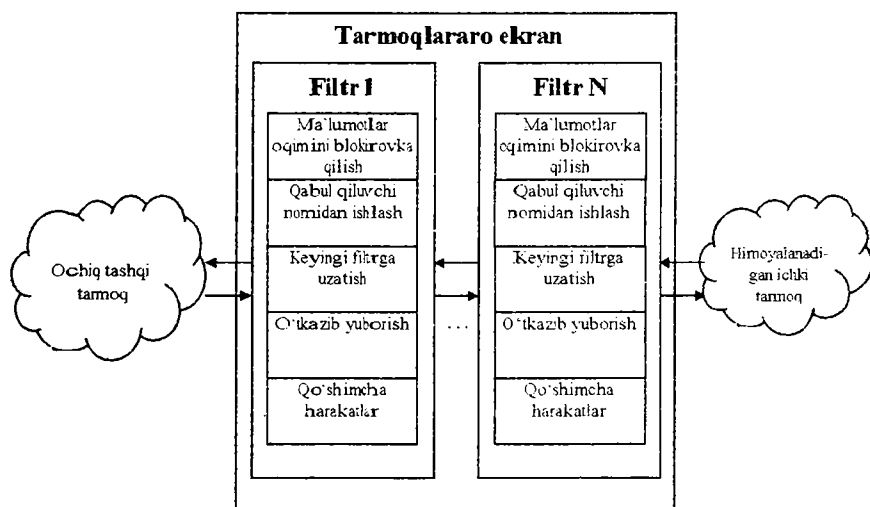
8.2-rasm. Tarmoqlararo ekran tuzilmasi.
