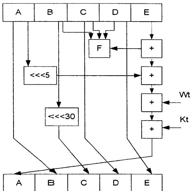
5.17-rasm. SHA-1 algoritmidagi bir iteratsiyasining sxemasi.
