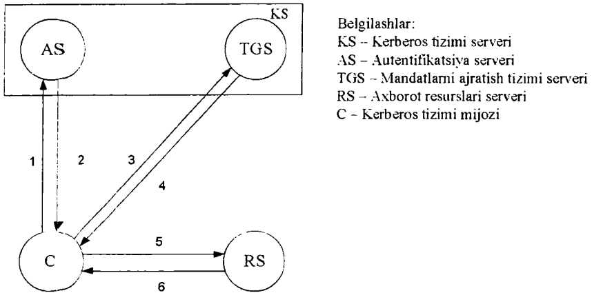
6.2-rasm. Kerberos protokolining ishlash sxemasi.
