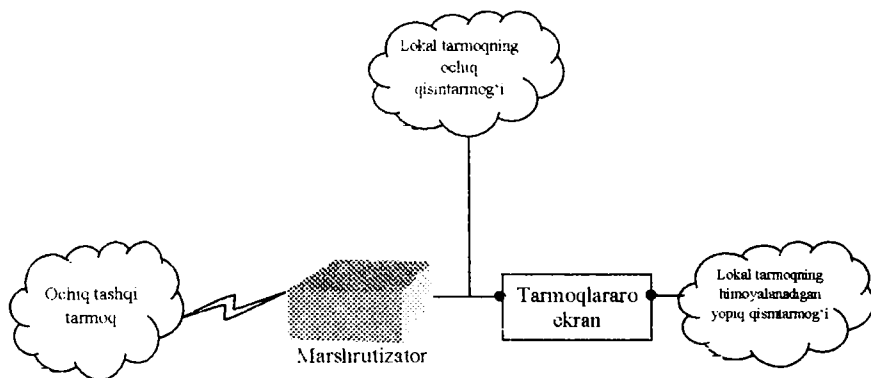
8.13-rasm. Himoyaladigan yopiq va himoyalamaydigan ochiq qismtarmoqli sxema.
