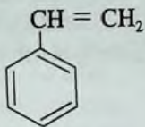
stirol, vinilbenzol, feniletilen
