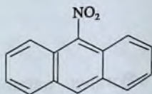
\gamma - nitroanratsen
