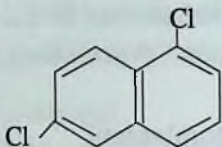
epi - dixlor- naftalin
