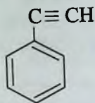
etinilbenzol, fenilatsetilen
