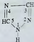
1, 2, 4 - triazol
