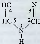
oksazol
