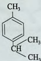
simol, 1-metil - 4- izopropilbenzol
