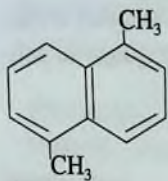
ana- dimetil- naftalin
