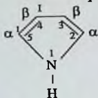
pirrol
