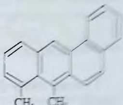
5,10-dimetil-1,2- benzantratsen
