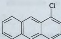
\alpha - xloranratsen
