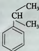
kumol, izopropilbenzol
