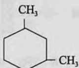
1,3 -dimetil-siklogeksan
