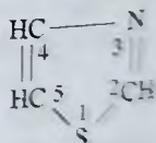
1, 2, 4 - triazol
