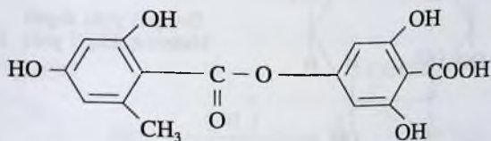
lekanor kislota
