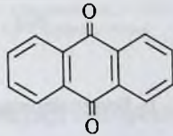
9,10-antraxinon
