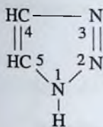
1, 2, 3 - triazol
