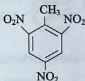
2,4,6 - trinitrotoluol
