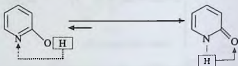
laktim shakli
