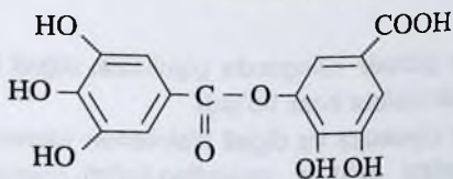
m – digall kislota
