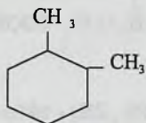
1,2-dimetil-siklogeksan
