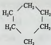
geksametilen
