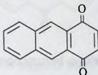
1,4-antraxinon
