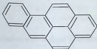
1,2 - benzpiren
