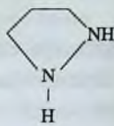
pirazolidin
