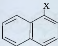
\alpha - izomer
