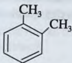
o – ksilol , o-dimetilbenzol, 1,2-dimetilbenzol
