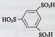
simm-benzoltrisulfokislota
