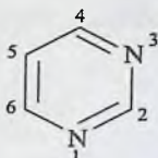
pirimidin (1,3 - diazin)
