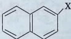
\beta - izomer
