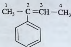
2-fenil-2-buten
