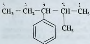
2-metil-3-fenilpentan
