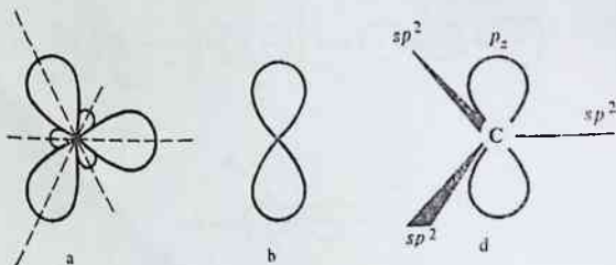
30-rasm. Alkenlarda C atomining ikkinchi valent holatini namoyon qiluvchi sp^2 -gibrid orbitallarining tuzilishi.
