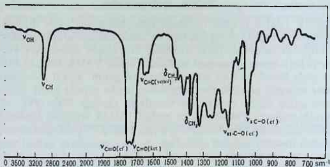
7-rasm. Metiletilketonning IQ spektri.
