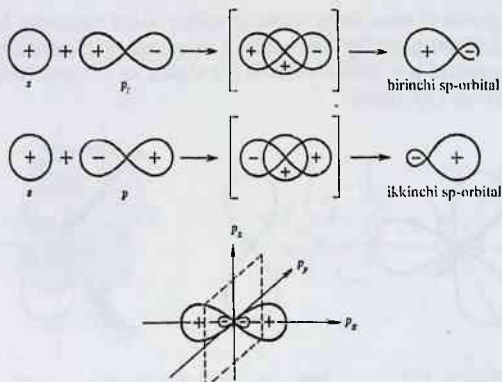
28-rasm. Uglerod atomidagi 1 ta s- va 1 ta p-orbitallarining gibridlanishi.
