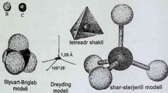
29-rasm. Metan molekulasining fazoviy tuzilishi.
