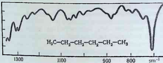
6-rasm. n-geksanning IQ spektri.
