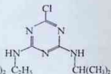
atrazin
