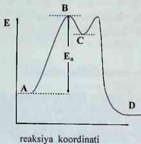
35-rasm. S_N1 -mexanizmli reaksiyaning energetik diagrammasi.
