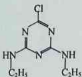
2-xlor-4,6-bis(etilami- no)-simm-triazin (simazin)
