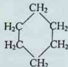
siklogeksan (geksametilen)
