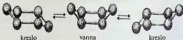
33-rasm. Siklogeksanning “vanna”, “kreslo” - konfiguratsiyalari va ularning bir-biriga o'tishi.
