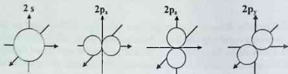
22-rasm. Uglrodning atom orbitalari.
