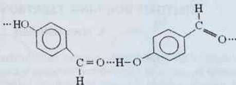
para-oksibenzaldegid
