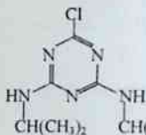
propazin
