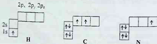
23-rasm. Atom orbitalida elektronlarning joylashish tartibi.
