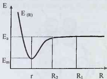
24-rasm. Vodorod molekulasining potensial energiya egri chizig'i.
