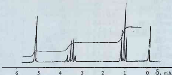
10-rasm. Etil spirtining PMR spektri.
