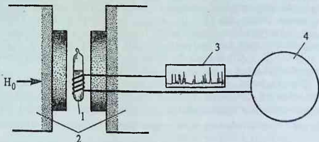
9-rasm. PMR spektri olishning oddiy ko'rinishi.
