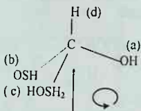
R- glitserin aldegidi
