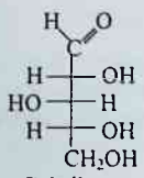
D-ksiloza
