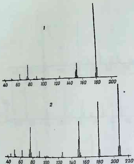
20-rasm. Intensivligi bir-biriga yaqin bo'lgan fluorenon – (1) va antraxinonlarning – (2) mass-spektrlari.
