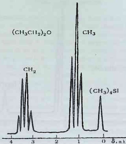
11-rasm. Dietil efrining PMR spektri.
