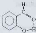
salitsil aldegid
