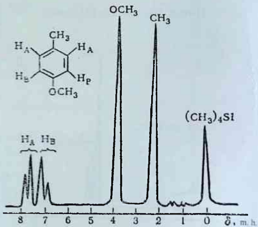
14-rasm. 4-metoksitoluolning PMR spektri.
