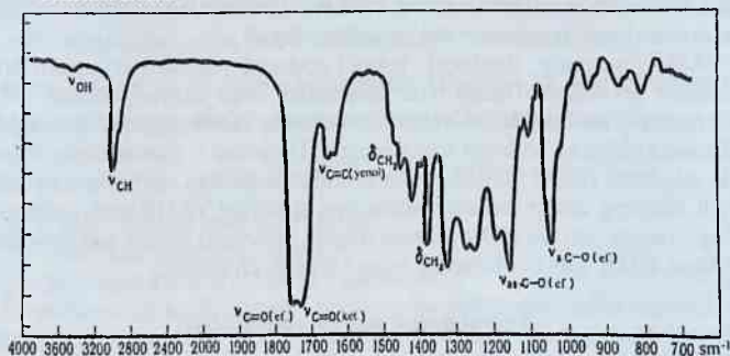
8-rasm. Atsetosirka kislota etil efirining IQ spektri.
