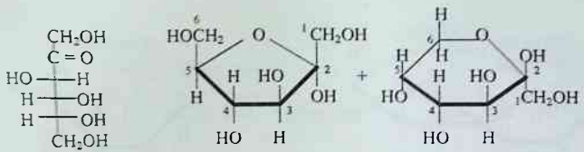
D-fruktoza \alpha -D(-)-fruktofuranoza \beta -D(-)-fruktopiranoza
