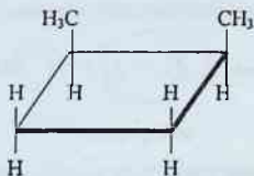
sis-1,2-dimetilsiklobutan
