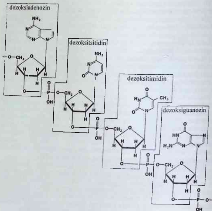
43-rasm. DNK molekulasining bir qismi: har qaysi ajratilgan fragment nukleozid bo'lib, unda asos bilan poliefir zanjirining o'zaro bog'lanishiga e'tibor bering.
