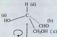
S- glitserin aldegidi
