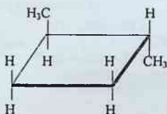
trans-1,2-dimetilsiklobutan
