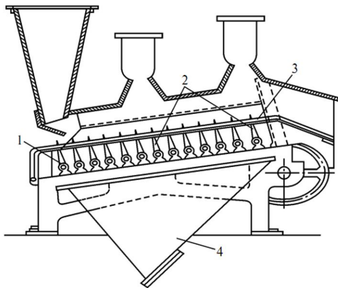
33-rasm. ТГ-135Л silkish dastgohi sxemasi.
