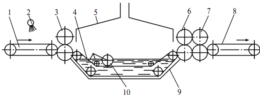
23-rasm. OPII-2MC siqish-yuvish mashinasining texnologik sxemasi.
