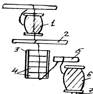
9.7-rasm. ChM-140-ShL dastgohi: 1-g`altak, 2-yo`naltiruvchi ko`zcha, 3-taraglash qurilmasi, 4-tozalash valiklari, 5- taxlagich, 6-tozalangan ip g`altagi, 7-urchuq.
