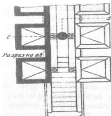
19-рasm. Yangi Aleksandriya qishloq xo'jalik institutidagi beton lizimetrylarning vertikal va gorizonta kelib ko'inishi.
