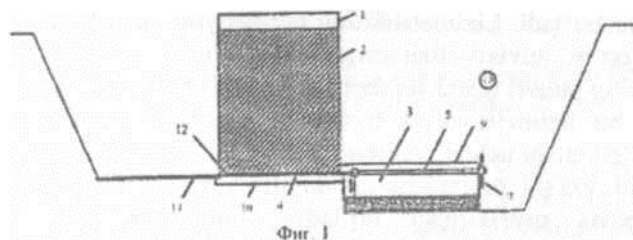
18-rasm. Melioratsiyaga oid tajribalar olib boriladigan lizimetr 1- lizimetrning yuqori tuproqsiz qismi, 2-tuproqli katlam, 3- filtr qatlam, 4- pastki shlak va shag'al yotkiziladigan qatlam, 5-suv sizib o'tadigan truba
