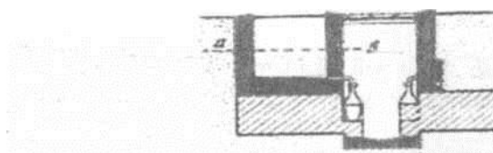
19-рasm. Yangi Aleksandriya qishloq xo'jalik institutidagi beton lizimetrylarning vertikal va gorizonta kelib ko'inishi.
