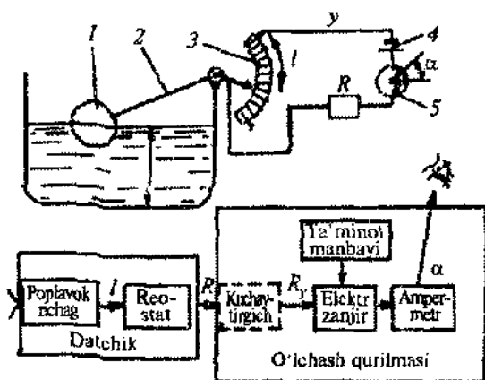
5.2-rasm. O'lanayotgan kattalikni bir turdan boshqa turga aylantirish (o'zgartirish) sxemasi.
