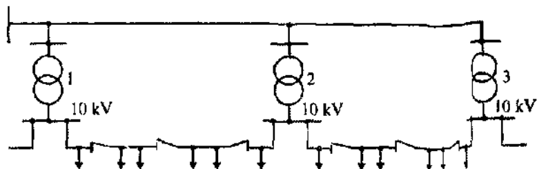
6.3-rasm. Ikki tomonlama energiya manbayiga ulangan elektr tarmoq'i sxemasi.
