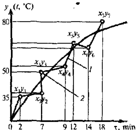
7.3-rasm. Asinxron dvigatel statori qizish egri chizig'i grafigi: 1 — bevosita o'lchamlar natijasi bo'yicha chizilgan egri chiziq; 2 — aproksiyalovchi bir maromdagi egri chiziq.
