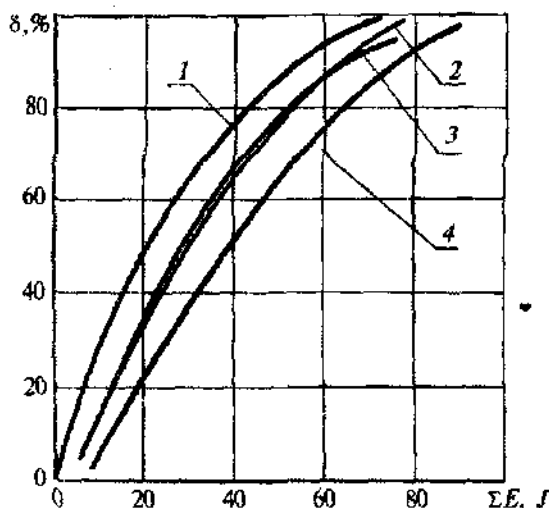
7.9-rasm. Uzun mevasi to'qimalari jonsizlanishi ( \delta ) unga kiritilayotgan umumiy energiya miqdoriga bog'liqligi.
