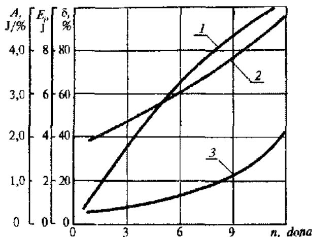
7.8-rasm. Razryad kuchlanishi va kondensator sig'imi optimal bo'lganda ( U_{opt} va C_{opt} ) uzum mevasi to'qimalari jonsizlanishi \delta (1-grafik), bitta impuls energiyasi E_i (2-grafik) va solishtirma energiyasi A (3-grafik)larning elektr razryadli impulslari soniga bog'liqligi grafiklari.
