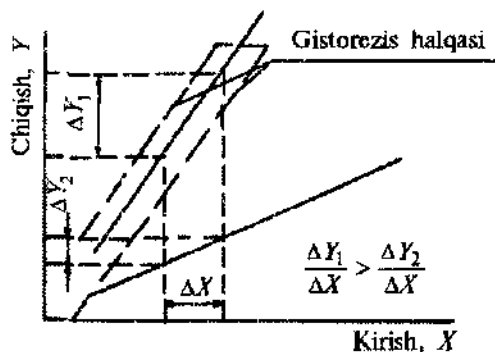
5.3-rasm. O'zgartirgichni (datchik)ning sezgirlikni tushuntirishga oid sxema.
