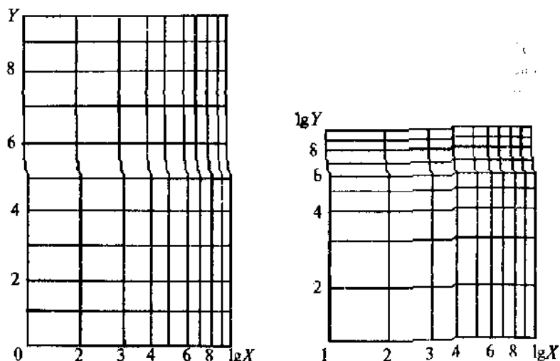
7.4-rasm. Yarimlogarifimik (a) va logarifimik (b) koordinata to'rlari.
