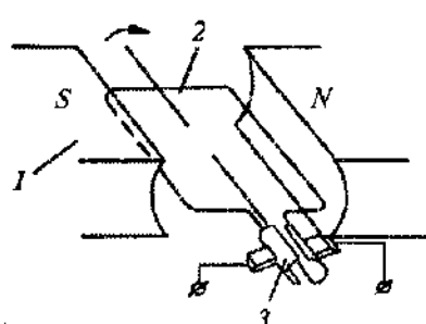
5.10-rasm. Induksion o'zgartirgich sxemasi (taxogenerator).
