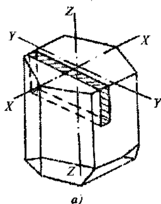
5.9-rasm. Pyzelektrik o'zgartirgichlar: a) pyezokristall (kvars kristali); b) probka tipidagi bosim datchigi.
