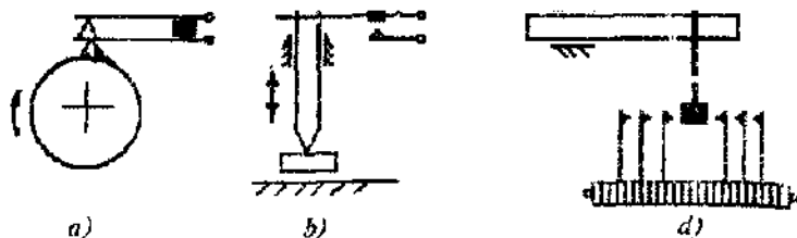
5.7-rasm. Kontaktli o'zgartirgichlar: a) bir kontaktli (valni aylanish chastotasini o'lash uchun); b) ikki kontaktli; d) ko'p kontaktli.
