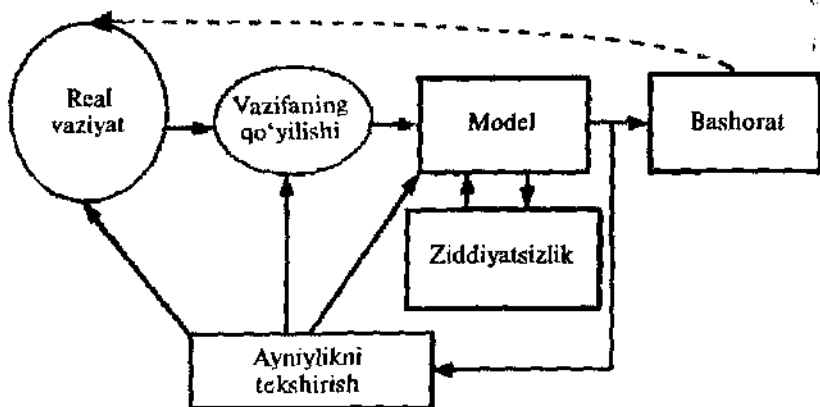
3.1-rasm. Matematik model ishlab chiqish tarxi.
