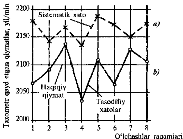
5.18-rasm. Taxometrli o'lchash qurilmasidan olingan xatoliklarning ko'rinishi.
