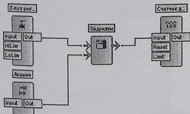
Рисунок 2.40. Функциональная блок схема с подключением объекта управление.
