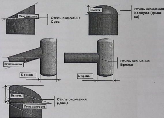
Рисунок 2.23 Параметры изменение 3D объектов в Master SCADA
