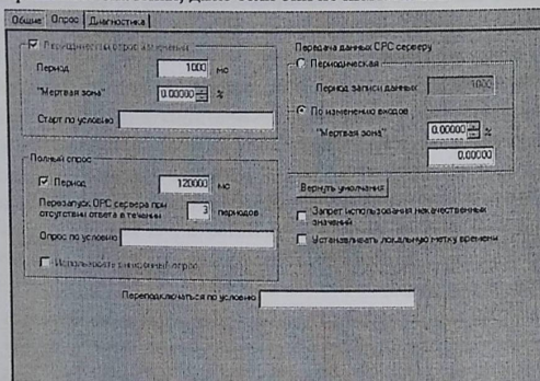
Рисунок 3.5. Общие параметры OPC
