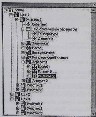
Рисунок 2.1. структура иерархия в Master SCADA
