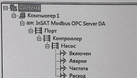
Рисунок 2.41. Дерево системы с OPC-сервером
