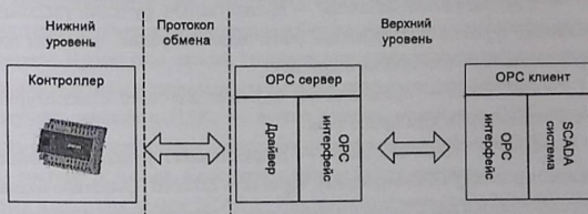
Рисунок 3.2. Функциональная связь через OPC-сервер
