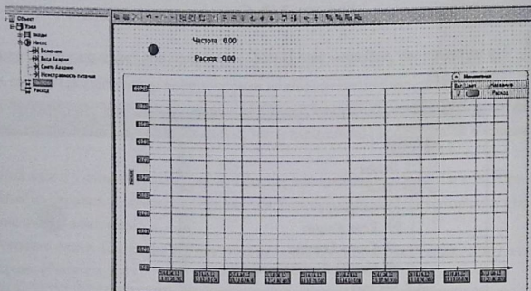
Рисунок 2.53. Готовая мнемосхема
