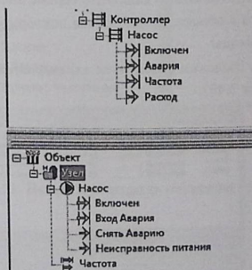
Рисунок 2.47. Создание значения частоты
