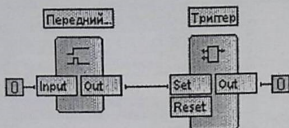
Рисунок 2.39. Функциональная блок схема.
