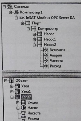
Рисунок 2.55. Дублирование объектов
