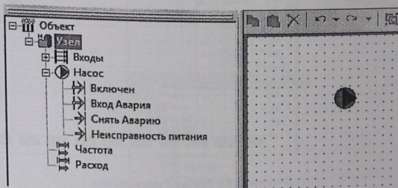
Рисунок 2.51. Вставка контрола насоса на мнемосхему
