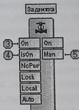
Рисунок 2.40. Функциональная блок исполнительного механизма.
