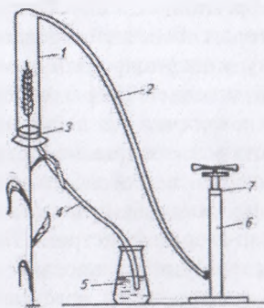
Рисунок 6 - Аппарат для инокуляции пшеницы и ячменя спорами пыльной головни (по Кривченко, 1985): 1 — стеклянный цилиндр; 2 — трубка для откачивания воздуха; 3 — вакуумная зажимная пробка; 4 — шланг для подачи суспензии спор; 5 — сосуд для суспензии спор; 6 — насос; 7 — резиновое кольцо
