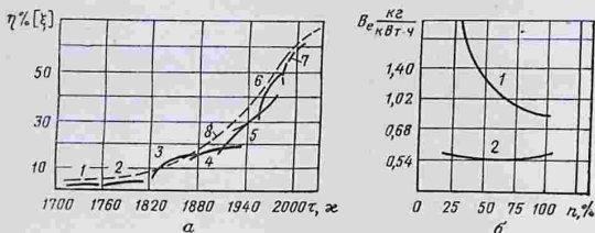
Рис. 8. Законы развития а и законы функционирования б техники. а : 1 — паровые машины Сэвери—Ньюкомена; 2 — паровые машины Уатта; 3 — усовершенствованные паровые машины; 4 — паровые машины с тройным расширением пара; 5 — первые паровые турбины; 6 — двигатели внутреннего сгорания (поршневые); паровые турбины высокого давления; 7 — топливные элементы; магнитогазодинамические электрогенераторные установки; 8 — оггибающая кривая;
