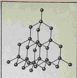
Рис. 75. Кристаллическая решетка алмаза. Кругами обозначены центры атомов углерода, черточками — ковалентные связи
