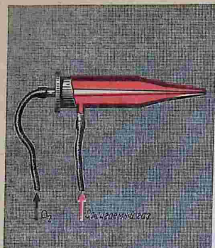
Рис. 21. Ацетилено-кислородная горелка (схема)
