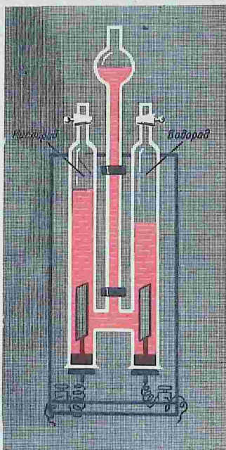
Рис. 8. Прибор для проведения электролиза воды
