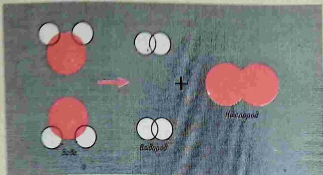
Рис. 9. Схема реакции разложения воды
