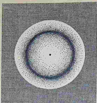
Рис. 65. Схема электронного облака атома водорода
