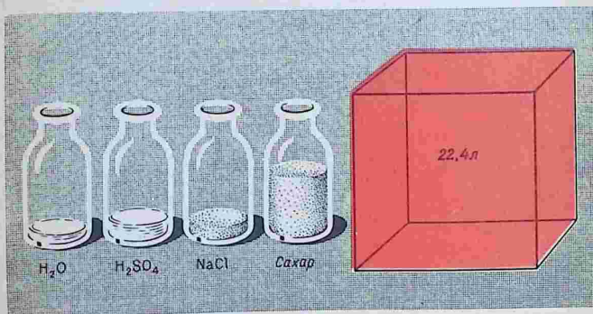
Рис. 81. Объемы разных веществ количеством вещества 1 моль
