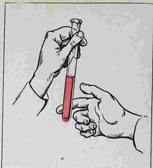
Рис. 53. Перемешивание жидкости в пробирке
