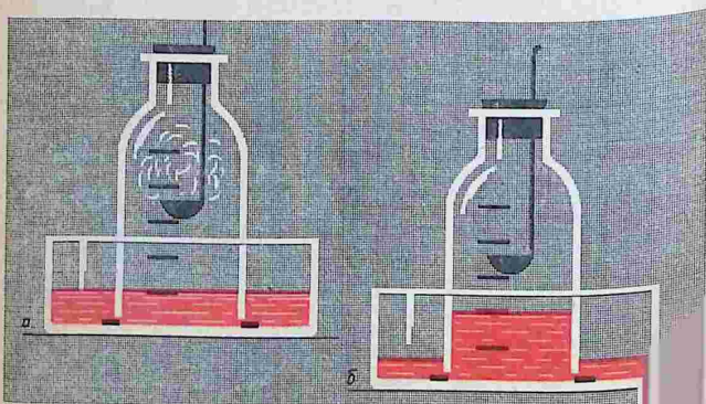
Рис. 26. Установление состава воздуха: а — прибор до опыта, б — прибор после опыта
