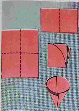
Рис. 61. Приготовление фильтра
