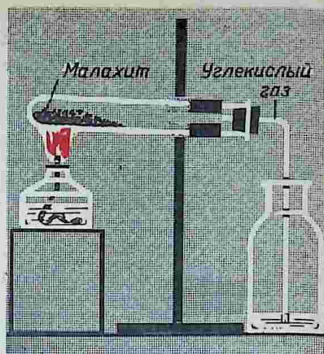
Рис. 13. Разложение малахита
