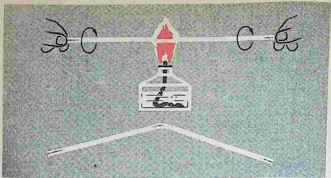
Рис. 54. Сгибание стеклянной трубки
