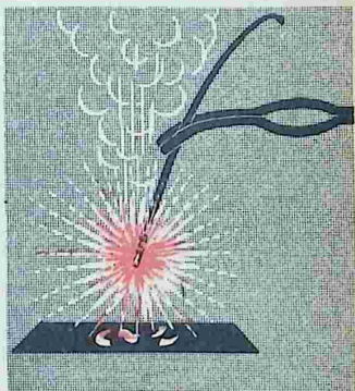
Рис. 4. Горение магния
