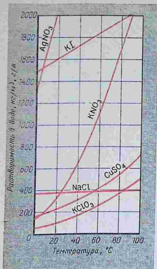
Рис. 46. Кривые растворимости некоторых солей
