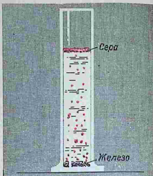
Рис. 1. Разделение смеси железа и серы: а — водой,
