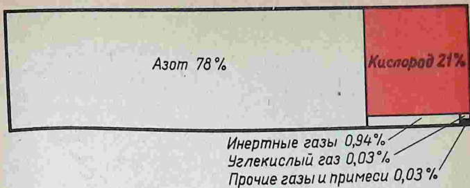
Рис. 27. Диаграмма объемного состава воздуха
