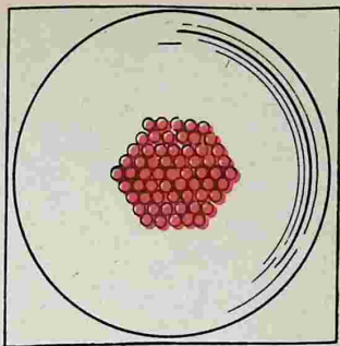
Рис. 71. Расположение горошин на блюдечке после встряхивания
