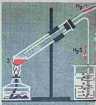
Рис. 89. Синтез сероводорода
