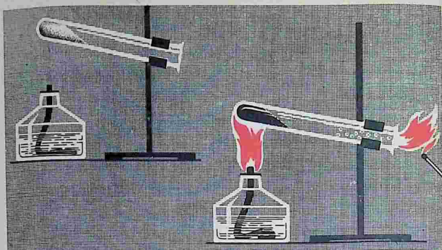
Рис. 5. Разложение сахара нагреванием
