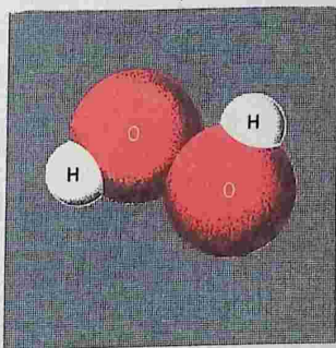
Рис. 70. Модель молекулы пероксида водорода
