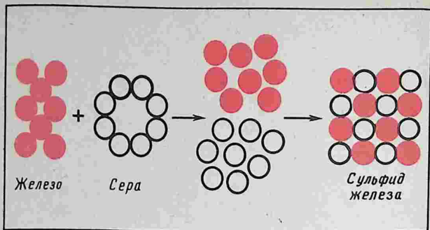
Рис. 11. Схема образования сульфида железа. Красными кружочками обозначены атомы железа, белыми — серы
