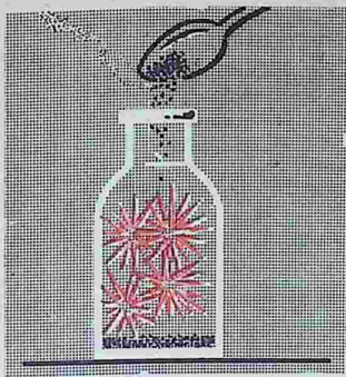
Рис. 76. Горение сурьмы в хлоре
