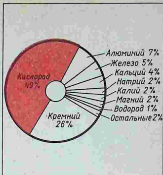
Рис. 15. Распространение атомов элементов в природе (по массе)
