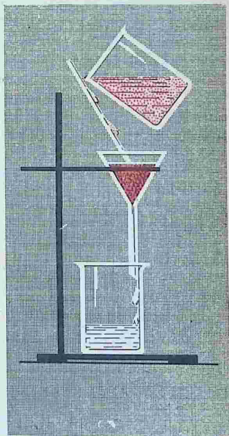
Рис. 2. Фильтрация
