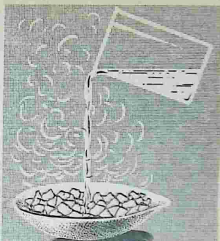
Рис. 49. Получение гидроксида кальция
