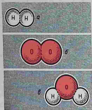
Рис. 7. Схема молекул водорода (а), кислорода (б) и воды (в)
