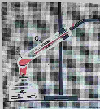
Рис. 88. Горение меди в парах серы
