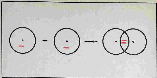
Рис. 67. Образование молекулы водорода из атомов
