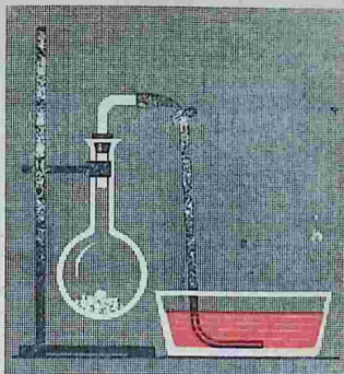
Рис. 51. Взаимодействие гидроксида натрия с углекислым газом
