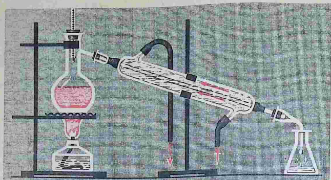
Рис. 42. Прибор для перегонки воды
