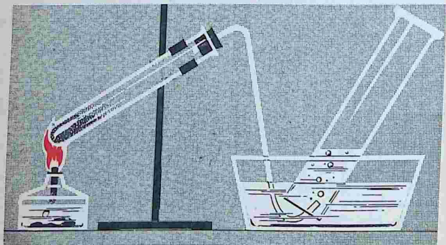
Рис. 23. Собиранье газа над водой
