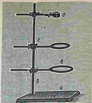
Рис. 60. Лабораторный штатив: а — подставка, б — стержень, в — кольцо, г — зажим, д — лапка
