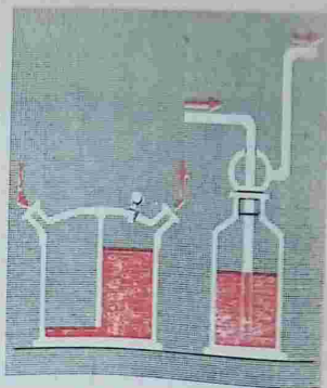
Рис. 91. Склянки для высушивания газов
