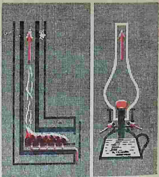
Рис. 30. Схема печи (а) и керосиновой лампы (б)
