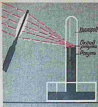
Рис. 14. Опыт Пристли
