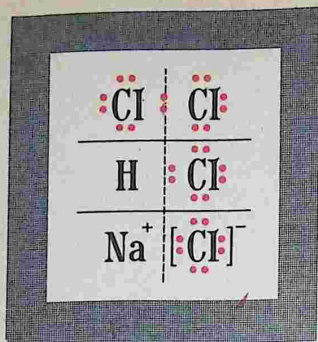
Рис. 69. Виды химической связи
