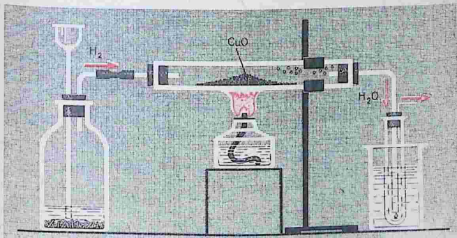
Рис. 39. Восстановление водородом меди из оксида меди (II)
