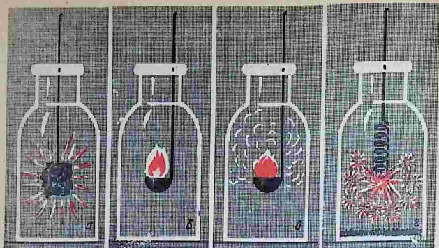
Рис. 16. Горение в кислороде: а — угля, б — серы, в — фосфора, г — железа
