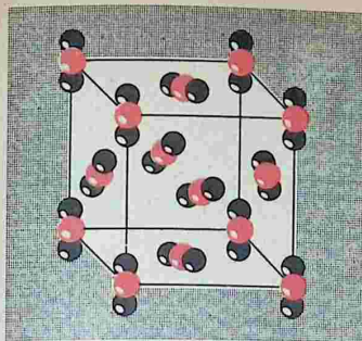
Рис. 74. Кристаллическая решетка твердого оксида углерода (IV)
