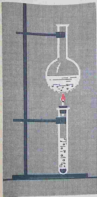
Рис. 90. Горение сероводорода с образованием воды
