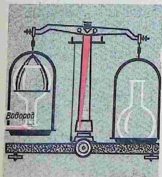
Рис. 33. Водород легче воздуха
