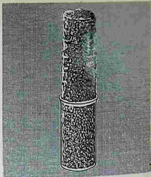
Рис. 92. Обугливание серной кислотой сахара
