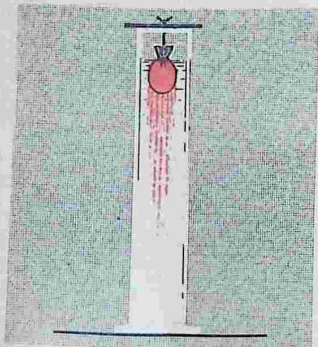
Рис. 44. Растворение медного купороса в воде
