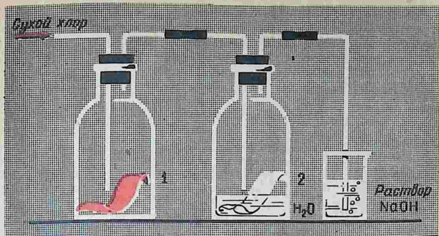
Рис. 80. Обесцвечивание хлором красящих веществ: 1 — сухая окрашенная ткань хлором не обесцвечивается, 2 — влажная ткань обесцвечивается
