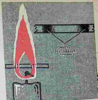
Рис. 19. Обугливание лучины в соответствующей части пламени
