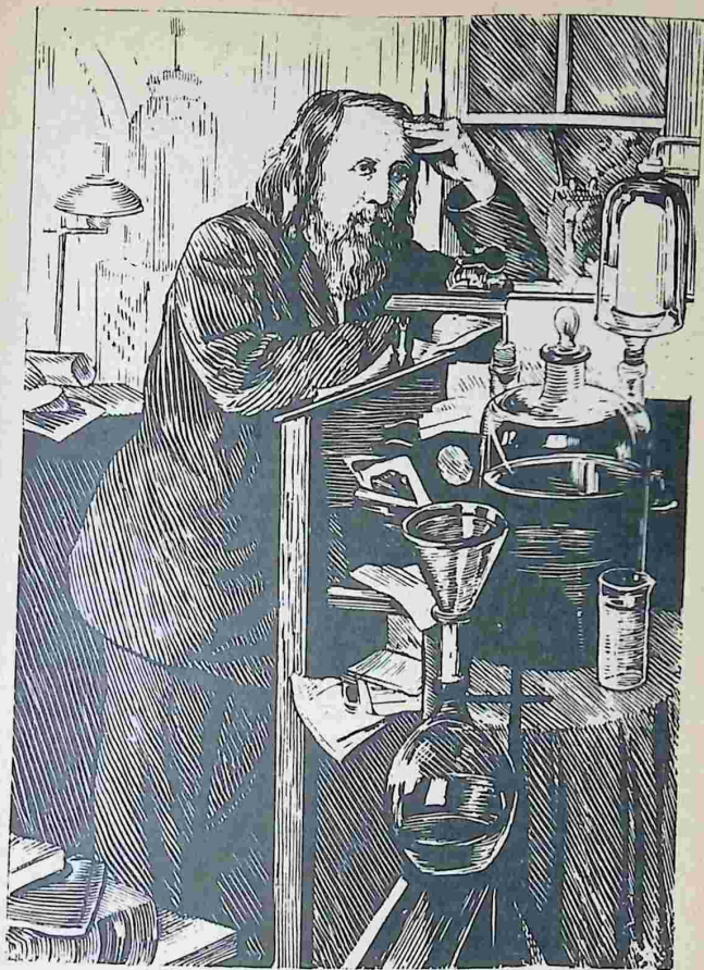
Дмитрий Иванович МЕНДЕЛЕЕВ (1834—1907)
