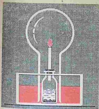
Рис. 40. Опыт Г. Кавендиша
