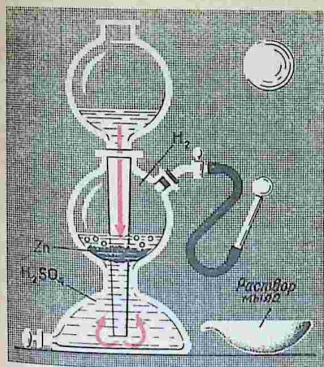
Рис. 34. Наполнение водородом мыльных пузырей
