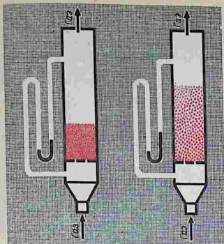
Рис. 96. Состояние слоя твердого материала при различных скоростях проходящего через него газа: а — слой с неподвижными частицами, б — «кипящий слой»
