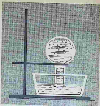
Рис. 79. Вытеснение кислорода хлором из воды
