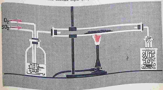
Рис. 94. Окисление оксида серы (IV) в присутствии катализатора
