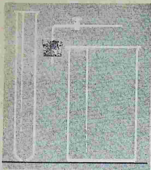
Рис. 32 Детали прибора для получения водорода
