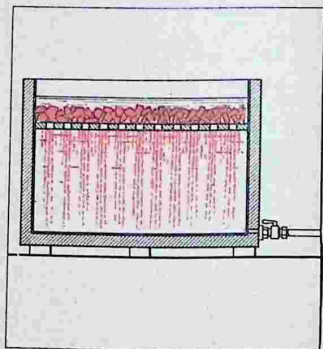
Рис. 45. Бак для растворения
