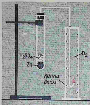
Рис. 36. Горение водорода в кислороде
