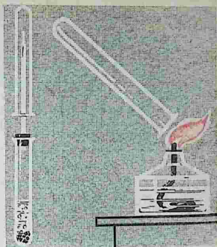
Рис. 38. Пробы водорода на чистоту
