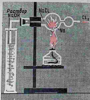
Рис. 63. Горение натрия в хлоре
