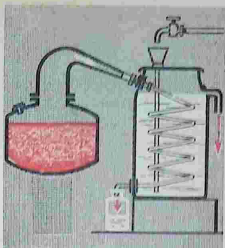
Рис. 43. Перегонный куб
