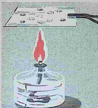
Рис. 55. Выпаривание капель раствора на стеклянной пластинке
