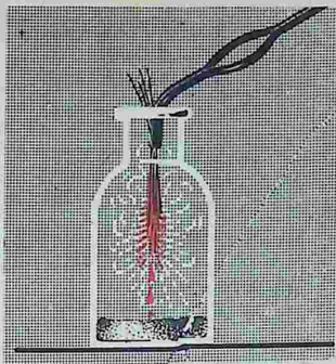
Рис. 77. Горение меди в хлоре
