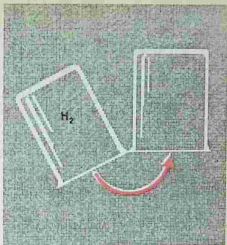
Рис. 35. Переливание водорода из сосуда в сосуд
