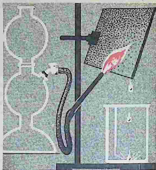
Рис. 37. Образование воды при горении водорода
