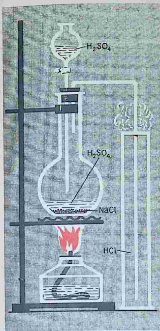
Рис. 84. Получение хлороводорода в лаборатории
