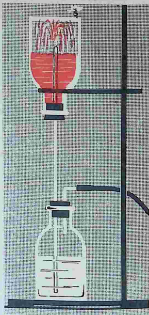
Рис. 85. Опыт, иллюстрирующий большую растворимость хлороводорода
