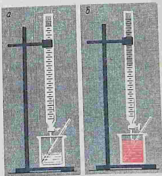
Рис. 50. Реакция нейтрализации
