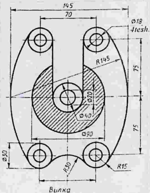
Вилка
