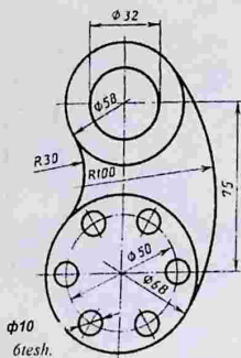
Кронштейн
