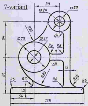
Станина
