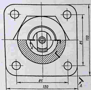
SAQLAGICH KLAPAN
