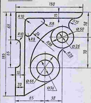
Кронштейн
