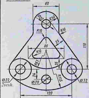
Подвеска
