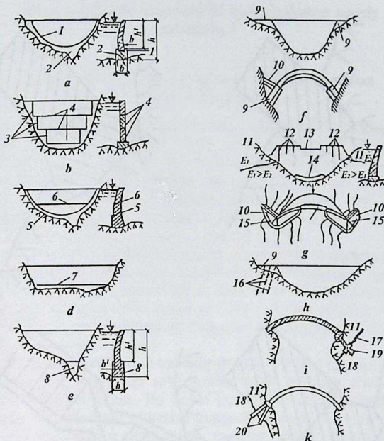
3.2- rasm. Arksimon to'g'onlarning sxemalari:
