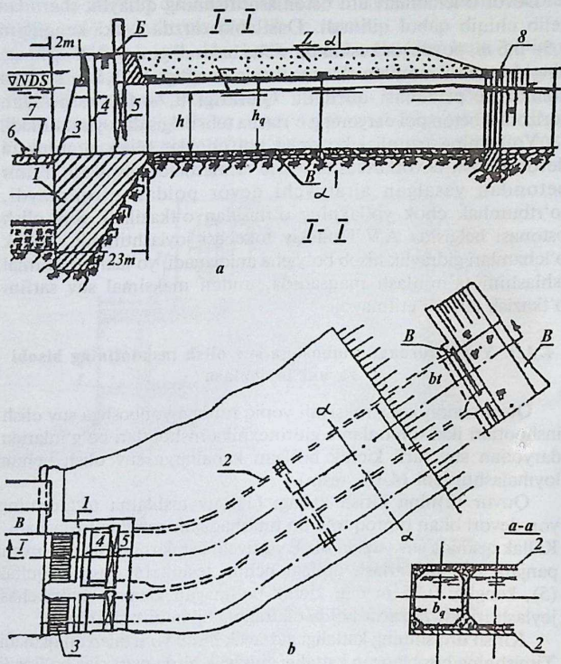
4.13- rasm. Yopiq turdagi yonboshdan suv olish inshootining konstruksiyasi: 1—kirish kallagi; 2—quvur; 3—panjara; 4—ta'mirlash qulfaklarining teshiklari; 5—asosiy qulfaklar; 6—suv tashlama to'g'onning ravoqlari; 7—A.V. Troiskiy tokchasi; 8—chiqish kallagi. I—I, II—II, — bo'ylama va ko'dalang kesimlar.
