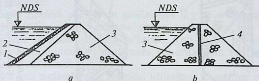
1.1- rasm. To'kmatosh to'g'onlarning turlari:
