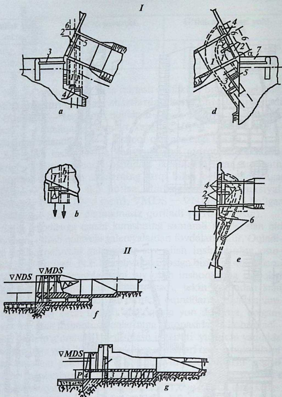
4.11- rasm. Oqindilarni ushlab qoluvchi galereyalarning konstruksiyasi:
