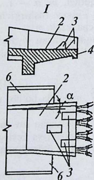
2.5- rasm. Konsolli sharsharak: 1—nov; 2—konsol; 3—trampinlar; 4—suv oqizma; 5—qirg'oq qoplamasi; 6—xizmat ko'prigi. I — konsolli sharsharakning chiqish qismining ko'rinishi.
