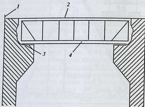
3.14- rasm. Kesikli bosim plitasining sxemasi:
