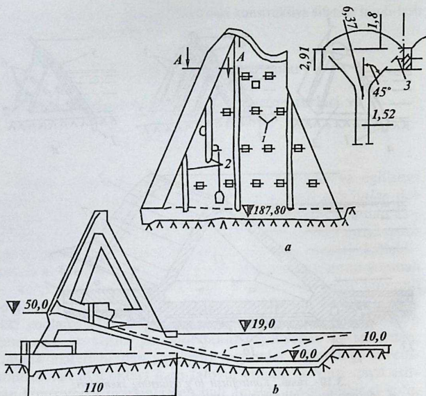
3.11- rasm. Suv tashlagichli massiv kontroforsli to'g'onlarning sxemalari: a—baland uchli suv tushirgichli to'g'on (Las—Virgenes, h = 47,6 m, Meksika); b—qo'sh kontroforslarida chuqurlikda oraliqlari bo'lgan to'g'on (Andijon, h = 115 m, O'zbekiston); 1—qattiqlik to'sini 1 \times 0,6 m; 2—vaqtinchalik ochiq choklar, kengligi 1,37 m; 3—mis list.
