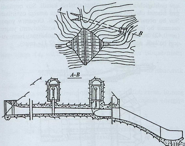
2.10- rasm. Tunelli suv tashlagich: A— B bo'ylama kesim.
