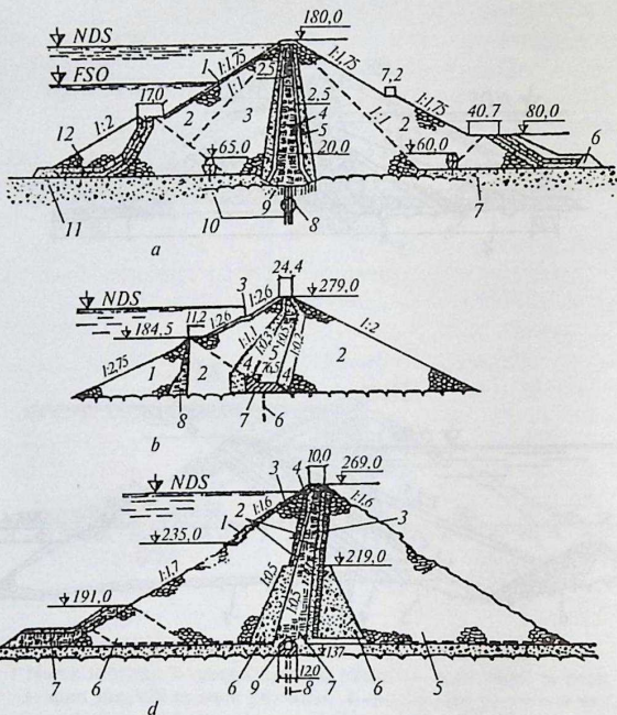
1.5- rasm. Yupqa gruntli o'zaklarga ega bo'lgan to'g'onlar:
