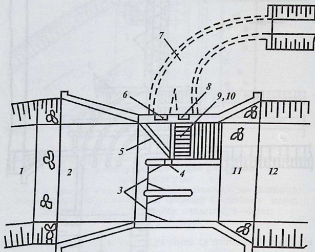
4.9- rasm. Ostli-panjarasimon gidrotexnika inshootlari bo'g'ini:
