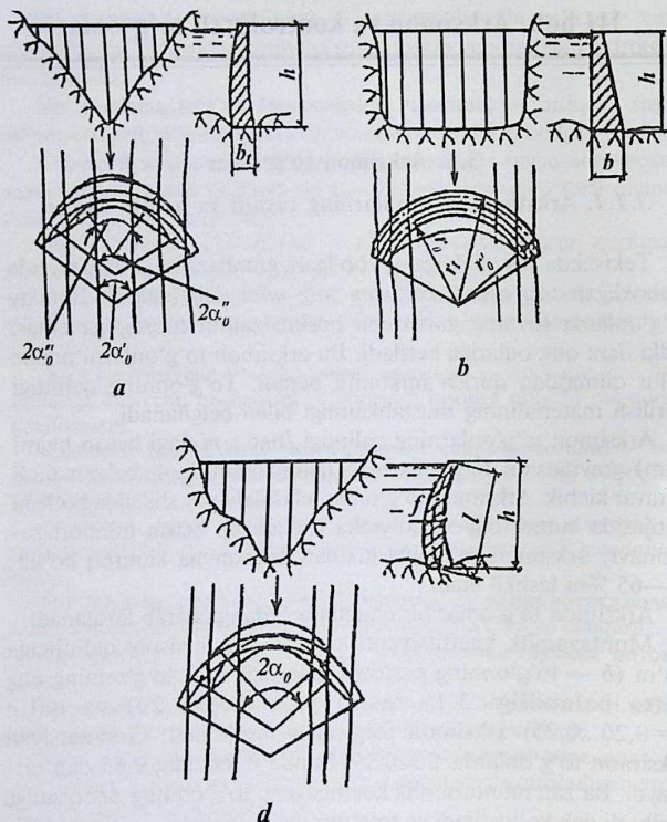
3.1- rasm. Arksimon to'g'onlarning turlari:
