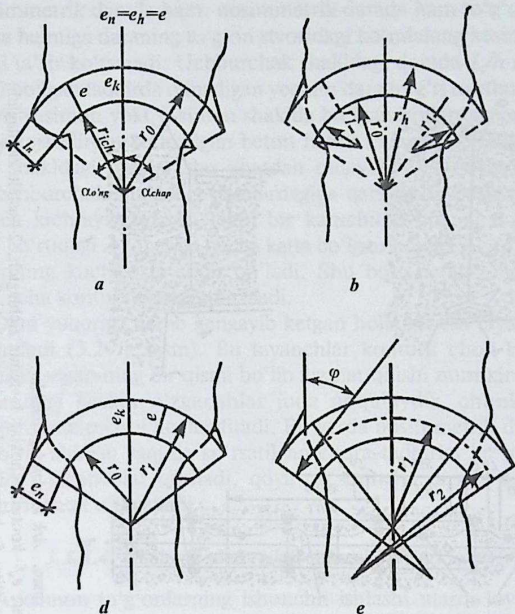
3.6- rasm. Ark halqalari sxemasi:
