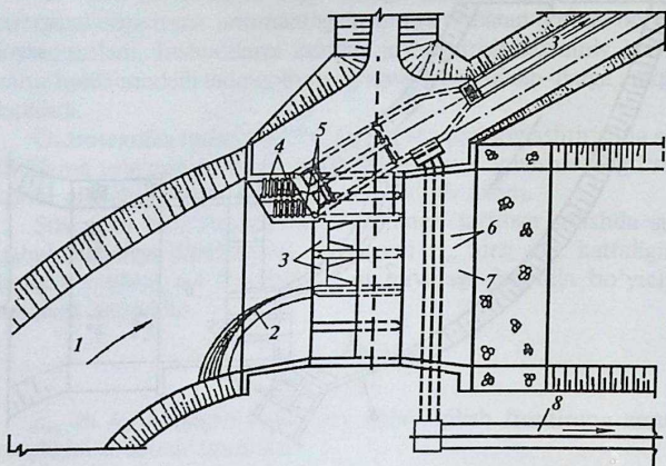
4.7- rasm. Oqimning ko'ndalang sirkulatsiyasidan foydalaniladigan hamda ejection yuvish galereyalari bo'lgan gidrotexnika inshootlari bo'g'ini:
