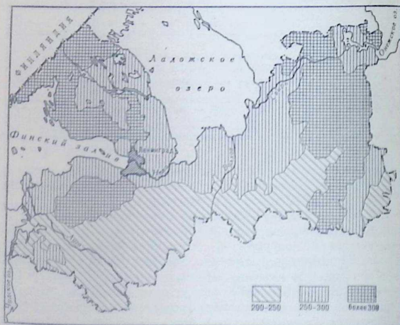
Рис. 21. Годовой слой стока по ландшафтам Ленинградской области (в мм)
