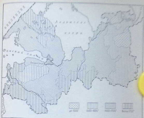
Рис. 16. Сумма температур за период со средними суточными температурами выше 10^{\circ} по ландшафтам Ленинградской области
