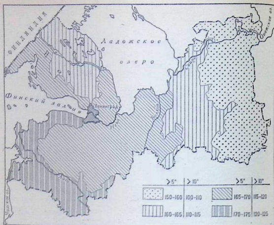
Рис. 17. Продолжительность периодов (число дней) со средними суточными температурами выше 5° и выше 10° по ландшафтам Ленинградской области
