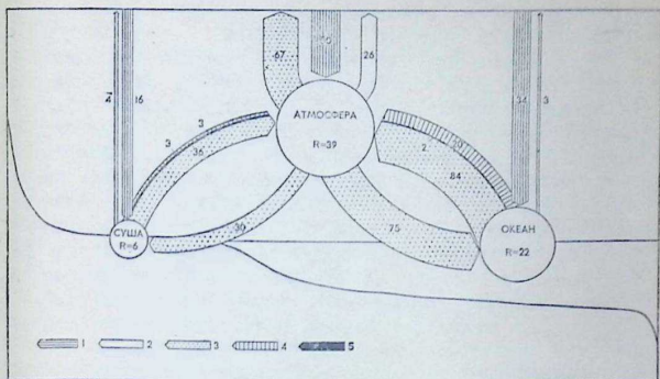
Рис. 6. Трансформация солнечной энергии в эпигеосфере:
