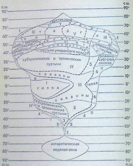
Рис. 9. Схема зонального и секторного деления суши (обобщенного материка).
