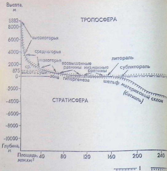
Рис. 5. Схема строения эпигеосферы
