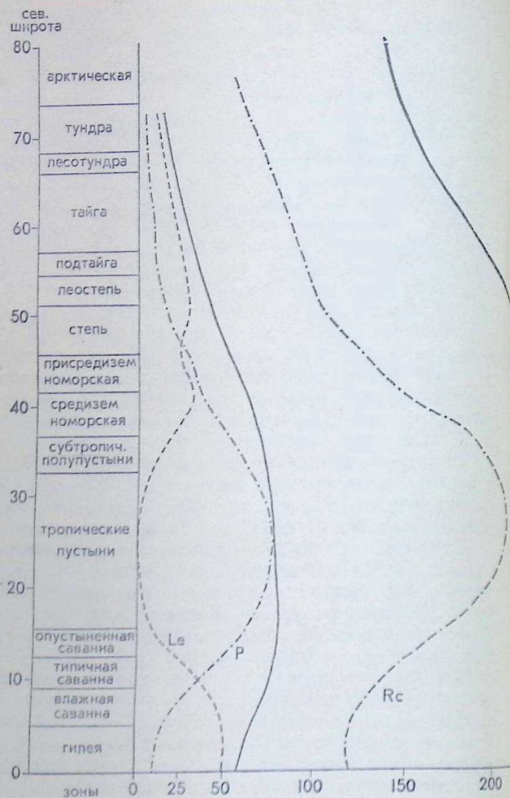
Рис. 7. Широтные изменения радиационного баланса и температуры воздуха (умеренно-континентальный сектор северного полушария): R_0 — солнечная радиация на верхней границе атмосферы, R_c — суммарная радиация у земной поверхности,
