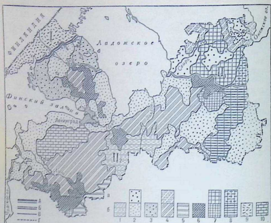
Рис. 13. Ландшафтная структура Ленинградской области
