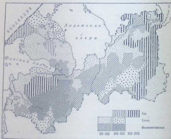
Рис. 23. Современные лесные ресурсы Ленинградской области. Преобладающие породы и общий средний запас древесины ( \text{м}^3/\text{га} ) по ландшафтам
