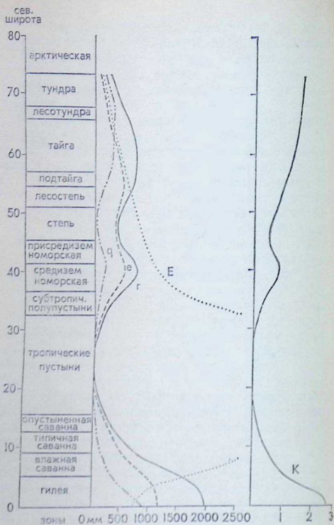
Рис. 8. Широтные изменения увлажнения и биологической продуктивности (для умеренно-континентального сектора северного полушария):
