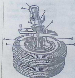
21-rasm. Tormoz barabanlarini silliglovchi va tormoz kolodkasining ishdan chiqqan qoplamalarini qiruvchi qo'zg'aluvchan moslama:
