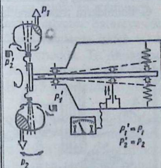
106-rasm. Qo'zg'almas muvozanatlash jihozining ishlash yo'rig'i:
