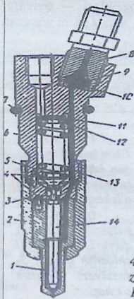
73-rasm. «KamAZ-740» dvigatelining forsunkasi
