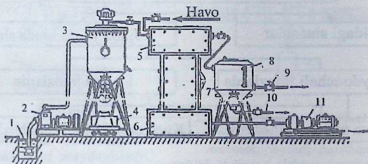
29-rasm. Suvdan qayta foydalanishda ishlatiladigan «KRISTALL» qurilmasi shakli
