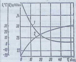
123-rasm. Agregatlarni qizdirish vaqtining, ularning boshlang'ich harorati va yonilg'i sarfiga ta'siri: 1- yonilg'i sarfi; 2- orqaga ko'priklar harorati
