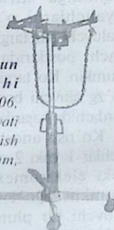
11-rasm. Harakatlanuvchi, yuk ko'tarish qobiliyati 20 tonnaga ega bo'lgan gidravlik domkrat (Markasi-5.8204, ko'tarish balandligi 220-680 mm, maydonchasi 179 mm, massasi 315 kg)
