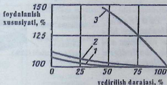
98-rasm. Protektor yedirilishining avtomobilning ekspluatatsiya xususiyatlariga ta'siri:
