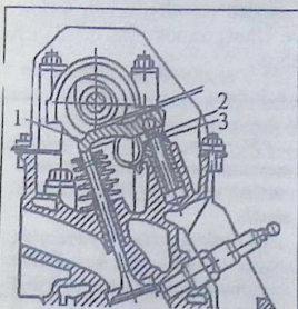
52-rasm. Klassik tuzilishdagi «VAZ», «Tiko» va «Matiz» avtomobillari gaz taqsimlash mexanizmining issiqlik tirqishini sozlash shakli.
