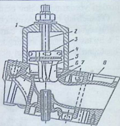
65-rasm. Klapan egarini joyiga qoqish shakli:
