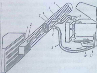
129-rasm. Avtomobil dvigatelni issiq suv yordamida o'toldirishdan avvalgi bir zunda isitishning prinsipial shakli:
