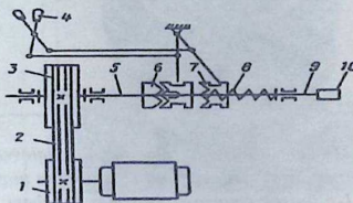
19-rasm. I330 modeli g'ildirak gaykasini qotirish va yechish gaykaburagichining prinsipial shakli:
