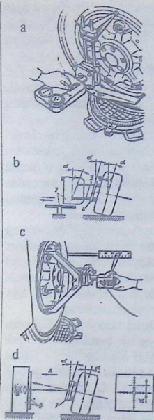
46-rasm. G'ildiraklarni statik tarzda nazorat qilish anjomlari: 1-shaytonli asbob; 2-yo'nalti-ruvchili o'lchash kallagi; 3-o'lchash sterjenlari; 4-g'ildirakka qoti-riluvchi tayanch disk; 5-proyektor; 5-o'lchash shkalasi bo'lgan nur tarqatish manbai; 6-ko'zguli nur qaytaruvchi
