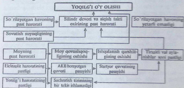
128-rasm. Dizel dvigatellarini o't oldirish vaqtida silindrdagi yonilg'ini alanganishiga ta'sir ko'rsatuvchi omillar
