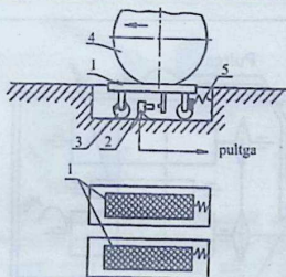
31-rasm. Tormozlarni tekshirishni maydonchali jihozining shakli
