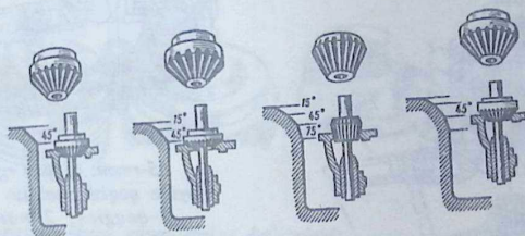
63-rasm. Klapan egarlarini yo'nish ketma-ketligi
