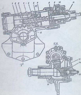
82-rasm. «ZIL-130» avtomobilining rul mexanizmi:
