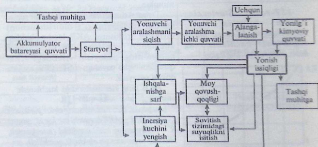
126-rasm. Dvigatelni ishga tushirishdagi akkumulyator quvvatini taqsimlanishi.
