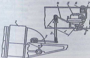
85-rasm. «ZIL-4331» avtomobilning tormoz kuchini sozlagichi:
