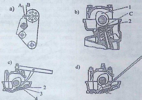
53-rasm. VAZ-2108 va VAZ-2109 turidagi avtomobillarining gaz taqsimlash mexanizmidagi issiqlik tirqishlarini sozlash ketma-ketligi:
