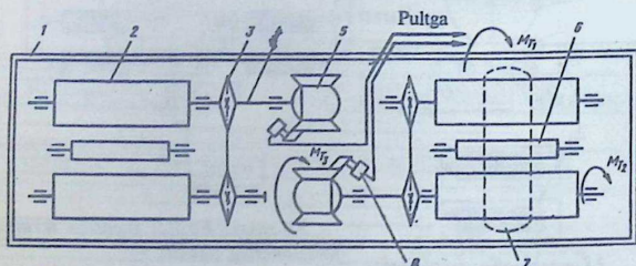
33-rasm. Kuchlar orqali ishlovchi rolikli tormoz jihozi shakli:
