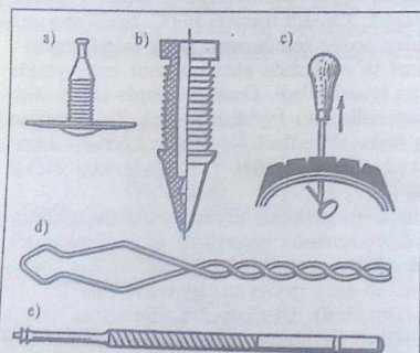
108-rasm. Shina teshiklarini ta'mirlash uchun moslama:
