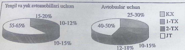
2-rasm. Avtomobillarni qayta tiklashgacha bo'lgan davr ichidagi TX va JT uchun sarflanadigan mehnat sarfi taqsimoti
