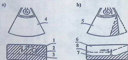
41 - r a s m . Simmetrik (a) va asimmetrik (b) yoritgichlarni tekshirish va sozlash shakli
