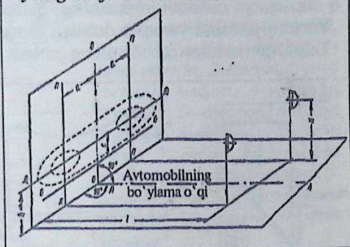
93-rasm. «Evropacha» assimetrik yorug'lik faralarini tekshirish.
