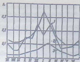
120-rasm. Ishdan chiqishlarning yil oylari bo'yicha taqsimlanishi: 1-dvigatel; 2-osma; 3-rul boshqarmasi.
