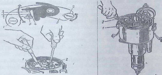
68-rasm. Uzgich kontaktleri sozlash(a) va tozalash(b): 1-kontaktlar, 2-abraziv plastana.
