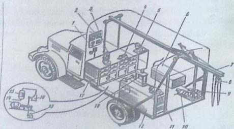
138-rasm. Harakatlanuvchi ta'mirlash ustaxonasi kuzovida jihozlarning joylashishi:
