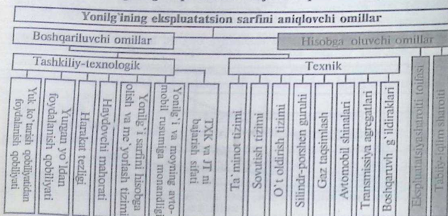
115-rasm. Yonilg'ining ekspluatatsion sarfini aniqlovchi asosiy omillar
