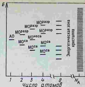
Рис. 4.14. Схема образования энергетической зоны кристалла лития
