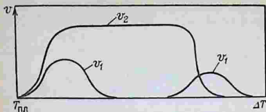
Рис. 5.4. Зависимость скорости образования зародышей v_1 и скорости роста кристалла v_2 в переохлажденной среде от температуры. \Delta T = T_{пл} - T
