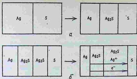
Рис. 5.13. Схема, иллюстрирующая механизм твердофазной реакции 2Ag + S = Ag_2S :
