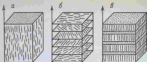
Рис. 4.7. Строение жидких кристаллов: а — нематических; б — холестерических; в — смектических
