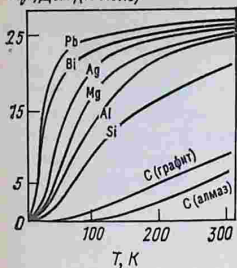
Рис. 4.8. Зависимость изохорной теплоемкости от температуры для простых кристаллических веществ
