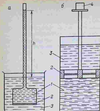
Рис. 3.11. Схема осмометра простейшей конструкции (а) и с поршнем (б).
