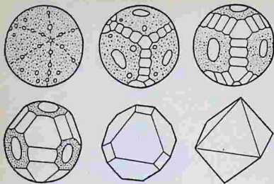
Рис. 5.7. Последовательность изменения формы кристалла в результате переноса вещества с быстро растущих граней на медленно растущие
