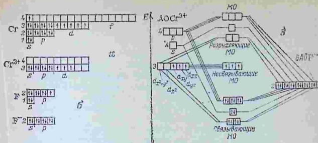
Рис. 4.27. Электронные конфигурации атома и иона хрома (а), атома и иона фтора (б) и энергетическая диаграмма молекулярных орбиталей иона [\text{CrF}_6]^{3-} (в)
