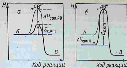
Рис. 3.20. Влияние соотношения энтальпий сольватации молекул исходных веществ и активного комплекса на энергию активации реакции A \rightarrow AB^* \rightarrow B :
