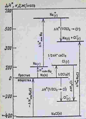
Рис. 4.28. Энтальпийная диаграмма перехода кристаллического хлорида натрия в изолированные ионы
