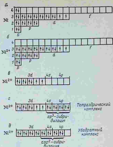
Рис. 4.21. Распределение электронов в атоме никеля (а), в изолированном ионе Ni^{2+} (б, в) и в ионах Ni^{2+} , входящих в тетраэдрический (г) и плоско-квадратный (д) комплексы
