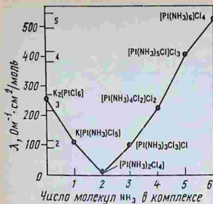
Рис. 3.22. Электропроводность растворов соединений платины (IV) в зависимости от их состава.
