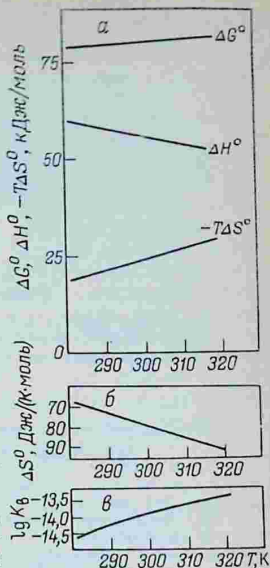
Рис. 3.5. Термодинамические характеристики \Delta G^\circ , \Delta H^\circ , -T\Delta S^\circ (а), \Delta S^\circ (б) и \lg K_w (в) электролитической диссоциации воды
