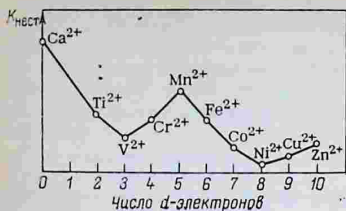
Рис. 6.4. Зависимость константы нестойкости комплексных ионов [M(H_2O)_6]^{2+} от числа d -электронов в атоме-комплекссообразователе
