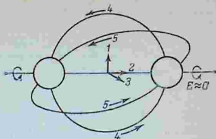
Рис. 2.1. Степени свободы движения двухатомной молекулы:
