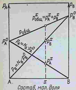
Рис. 3.9. Зависимость парциальных давлений пары компонентов p_A и p_B раствора и общего давления насыщенного пара p_{\text{общ}} над раствором от его состава
