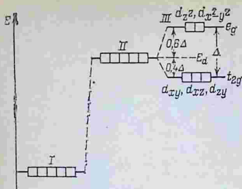
Рис. 4.23. Энергетическая диаграмма расщепления d -подуровня иона-комплексообразователя в октаэдрическом поле лигандов:
