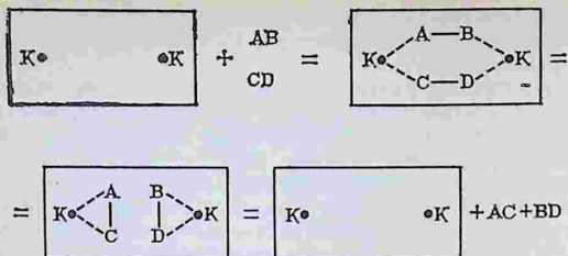
Рис. 5.2. Схема реакции AB + CD = AC + BD , протекающей на поверхности катализатора.
