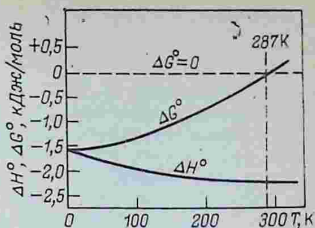
Рис. 4.31. Температурная зависимость изменения энтальпии \Delta H^\circ и изобарного потенциала \Delta G^\circ перехода графит→алмаз
