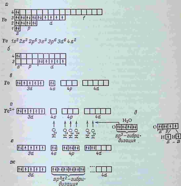
Рис. 3.23. Схема образования комплексного иона [\text{Fe}(\text{H}_2\text{O})_6]^{2+} по методу валентных связей;
