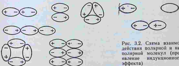
Рис. 3.1. Схема образования ассоциатов полярных молекул
