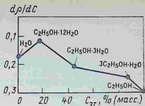
Рис. 3.7. Зависимость плотности ( d\rho/dC ) раствора от его состава для системы вода—этанол
