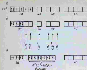
Рис. 3.24. Схема образования комплексного иона [Fe(CN)_6]^{4-} :
