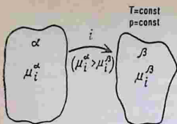
Рис. 1.2. Схема самопроизвольного перехода вещества i из одной фазы \alpha в другую \beta с различными химическими потенциалами
