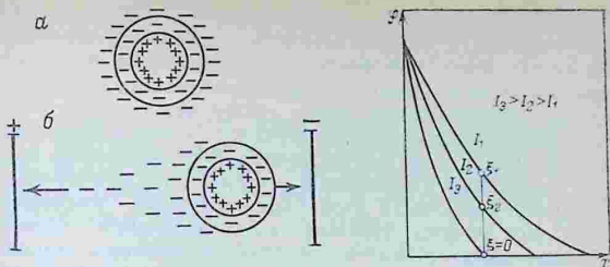
Рис. 3.32. Мицелла золя без воздействия внешнего электрического поля (а) и ее перемещение в электрическом поле (б)
