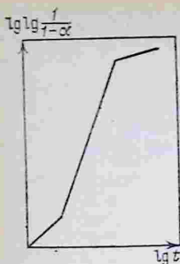
Рис. 4.36. Представление кинетической кривой «степень превращения вещества — время» в виде нескольких линейных зависимостей
