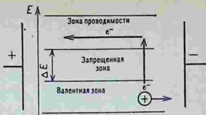
Рис. 4.17. Схема, характеризующая механизм собственной проводимости полупроводника
