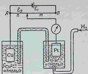
Рис. 5.10. Принципиальная схема водородного электрода
