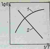
Рис. 4.19. Зависимость электропроводности металла (1) и полупроводника (2) от температуры
