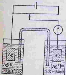
Рис. 5.12. Схема концентрационного элемента для измерения произведения растворимости бромида серебра
