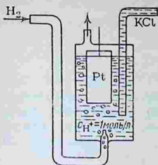
Рис. 5.10. Принципиальная схема водородного электрода
