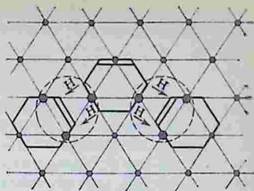
Рис. 5.3. Схема реакции 3C_6H_{10} = C_6H_6 + 2C_6H_{12} , протекающей на поверхности октаэдрической грани кристалла платины
