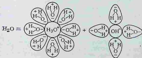
Рис. 3.6. Схема диссоциации воды
