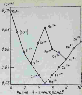
Рис. 4.26. Диаграмма ионных радиусов комплекссообразователей в ряду d -элементов четвертого периода с различным числом d -электронов
