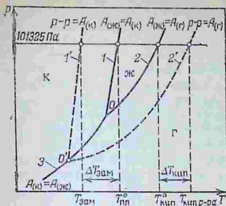
Рис. 3.14. Диаграмма состояния чистого растворителя А (1, 1', 3) и раствора (2, 2')
