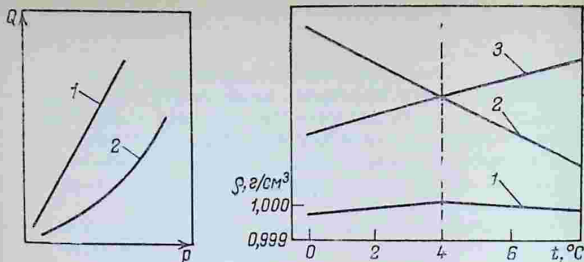
Рис. 3.3. Зависимость количества Q нормальной (1) и аномальной (2) жидкости, протекающей через капилляр, от давления
