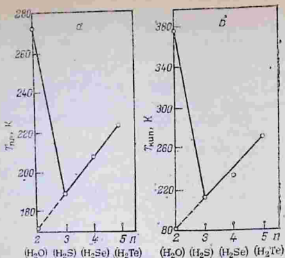
Рис. 1.7. Изменение температур плавления (а) и кипения (б) в ряду водородных соединений элементов VI группы
