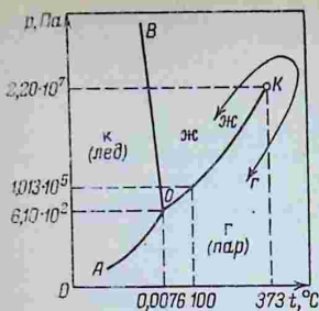
Рис. 1.6. Диаграмма состояния воды. Масштаб произвольный
