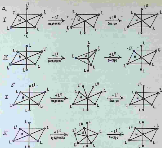
Рис. 6.7. Два возможных пути (I и II) протекания реакции замещения с участием октаэдрического комплекса [ML_5L^I] по диссоциативному (а) и ассоциативному (б) механизму
