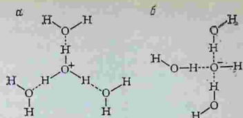
Рис. 3.18. Строение ионов \text{H}_3\text{O}_4^{3-} (а) и \text{H}_7\text{O}_4^{3-} (б)
