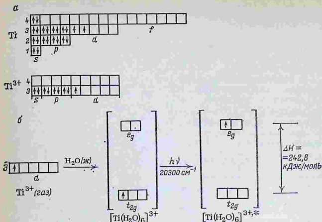
Рис. 6.6. Электронное строение атома Ti, иона Ti^{3+} (а) и схема электронного перехода в Ti^{3+} при поглощении видимого света водным раствором соли титана (б)
