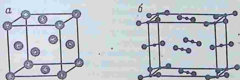
Рис. 4.4. Молекулярная решетка кристаллов аргона (а) и иода (б)
