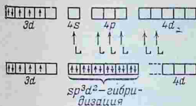
Рис. 3.25. Распределение электронов иона \text{Fe}^{3+} в окружении слабых и сильных лигандов
