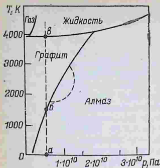
Рис. 4.30. Диаграмма состояния углерода:
