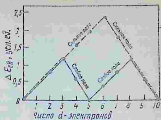
Рис. 4.24. Зависимость \Delta E_{\text{св}} октаэдрических комплексов в сильном и слабом полях лигандов от числа d -электронов иона-комплексобразователя
