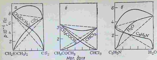
Рис. 3.10. Зависимость парциальных и общего давления пара над раствором от состава для систем, не подчиняющихся закону Рауля:
