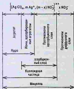
Рис. 3.30. Строение мицеллы золя хлорида серебра
