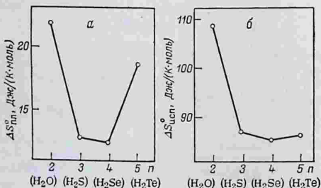
Рис. 1.9. Изменение энтропии плавления (а) и испарения (б) в ряду водородных соединений элементов VI группы
