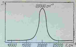
Рис. 6.5. Спектр поглощения водного раствора, содержащего Ti^{3+}
