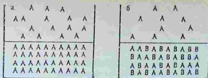
Рис. 3.8. Схема испарения чистого растворителя А (а) и растворителя из раствора, содержащего вещество В (б)
