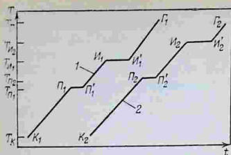
Рис. 1.5. Кривые нагревания при постоянном давлении p_1 (1) и p_2 (2); p_2 > p_1
