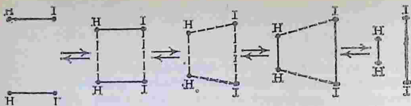
Рис. 2.6. Схема обратимой реакции образования и разложения иодоводорода. Сплошные линии между атомами означают прочные химические связи в молекуле, пунктирные — образующиеся или разрывающиеся связи
