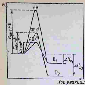
Рис. 2.7. Энтальпийная диаграмма реакций некаталитической A+B=D и с участием катализаторов K' и K''
