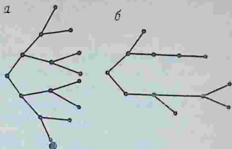
Рис. 2.4. Схема разветвленного цепного процесса (а) и процесса с редкоразветвленной цепью (б)
