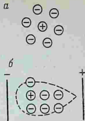
Рис. 6.1. Ионная оболочка вокруг катиона (а) и состояние катиона в электрическом поле (б)
