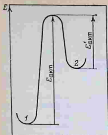
Рис. 4.12. Энергия активации образования дефекта по Френкелю:
