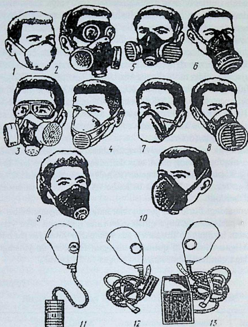
6.1-rasm. Nafas olish organlarini himoyalovchi respirator va gazniqoblar.
