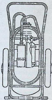
13.3-rasm. Qo'zg'aluvchi QXK -100 havo - ko'pikli o't o'chirgich
