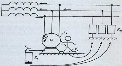
12.2 rasm. Himoyalovchi yerga ulashning ishlash chizmasi.
