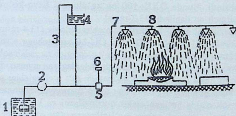
13.5-rasm. Sprinkler qurilmasining chizmasi.
