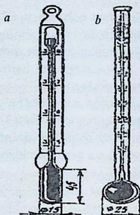
5.4-rasm. Katatermometrlar: a) silindrik; b) sharsimon.
