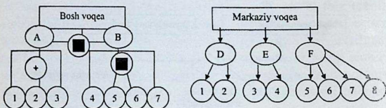
2.2-rasm. Hodisalar daraxti (1) va voqealar daraxti, uning natijalari (2).
