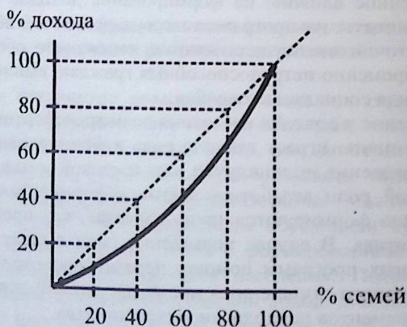
Рис. 1. Кривая Лоренца
