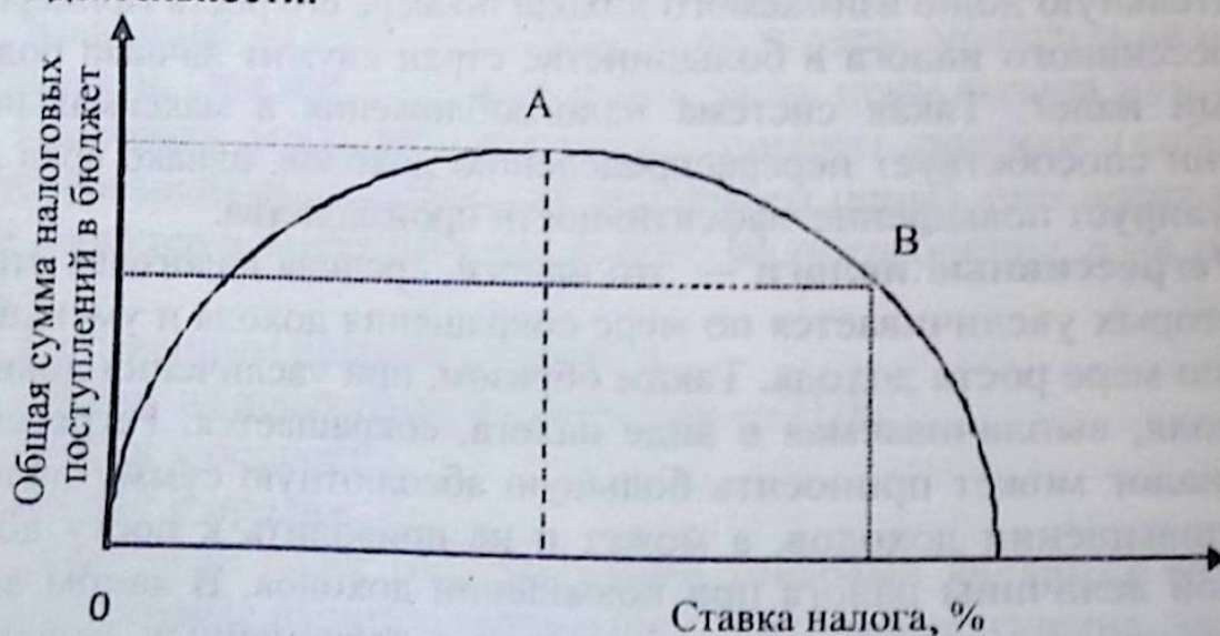
Рис. 1. Кривая Лаффера
