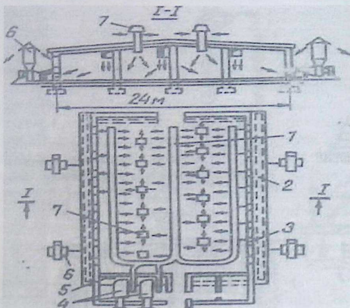
7-rasm. Parrandaxonalardag iyuqoridan - pastga ventilyasiyasining qurilmasi:
