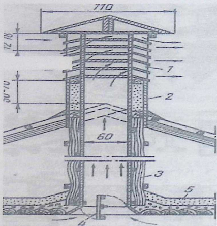
5-rasm. Havo chiqaruvchi quvur: 1 – deflektor. 2 - issiklikdan saqlovchi tekislangan quti. 3 - paxol qatlam. 4 – yopgʻich. 5 - isitish qatlami.
