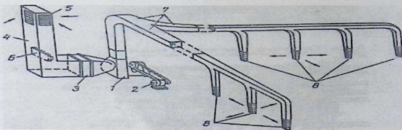
6 - rasm. Mexanik yoʻl bilan havoni qoʻzgʻatuvchi va isituvchi ventilyasiya qurilmasi: 1 - markazdan qochma ventilyator. 2 - elektromotor. 3 - kolorifer. 4 - tashqi havoga chiqaradigan shaxta. 5 - pardali panjara. 6 - klapan. 7 - havo yurish yoʻllari. 8 - havo kirish yoʻllari.
