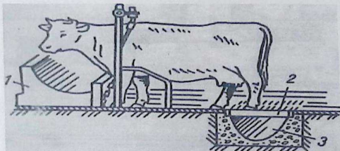
3-rasm. Signrxonada yoriq polning tuzilishi.
