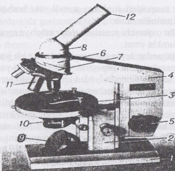
7-rasm. «Biolam» biologik mikroskopining tuzilishi:
