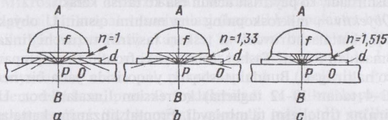
9-rasm. Optik mikroskopning obyektivi:
