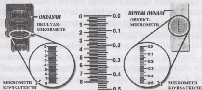
10-rasm. Obyekt-mikrometr va okulyar-mikrometr shkalasini taqqoslash 1 .
