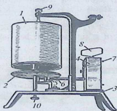
37-rasm. 1 – kimograf: 1 – baraban, 2 – disk, 3 – shtativ va unga o'rnatilgan 4 – soat mexanizmi, 5 – mufta, 6 – asos yoki o'q, 7 – uzatkich, 8 – flyuger, 9 – yuqori va 10 – pastki vint.
