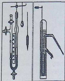
39-rasm. V simobli Manometr — Lyudvig manometri.
