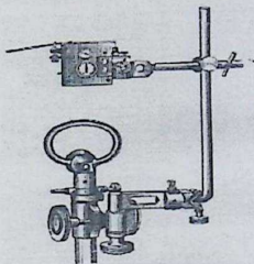
42-rasm. Jake xronografi.
