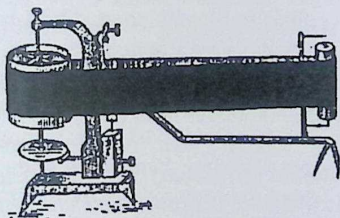
2 – barabanli kimograf.
