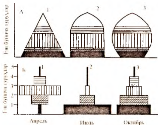
54-расм. Ҳайвонлар популяциясида ёш бўйича тузилиш. А— умумий схема; Б— моллюскалар популяциясининг турли-ёшли гуруҳларининг фасаллар бўйича ўзгаришин (Одум, 1975).
