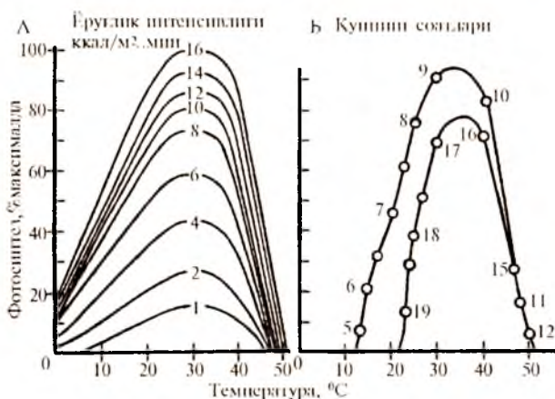
77-расм. Фотосинтез активлигининг барг ҳарорати ва нурунинг тушишига (А) боғлиқлиги. Фотосинтезнинг кун давомида ўзгариши (Б) (Реклефс буйича)
