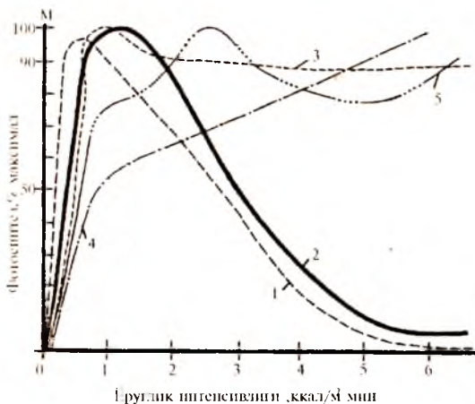
76-расм. Яшил (1), диатом (2) сувўтлари, эмон (3), қарагай (4) ва қизил (5) дарахтларда фотосинтез ва ёруғлик активлигини бир-бирига боғлиқлиги (Реклефе, 1979)
