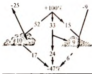
9-расм. Қисқа тўлқинли радиация кучининг атмосферадан ўтишида камайиши (Дажо, 1975).
