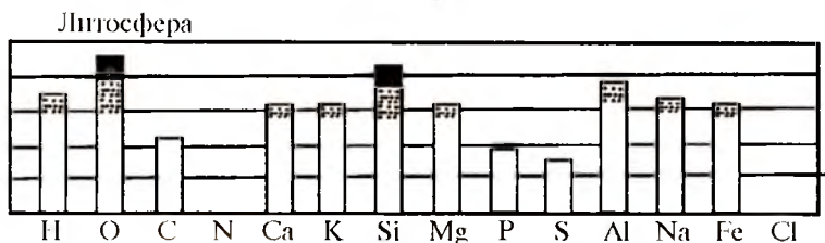
87-расм. Литосферанинг тузилишида ҳар хил кимёвий элементларнинг қатнашиши (Deevey, 1970)
