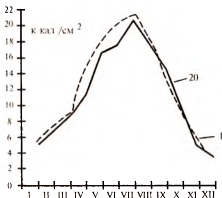
10-расм. Ўрта Осиёда қуёш радиациясининг ойлар бўйича миқдори, ккал/см². 1—1968 йил; 2—1988йил.
