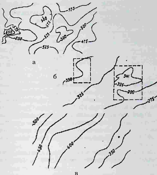
8.5.2.1 расм. Асосий (а), қисман (б) ва енгил (в) текисланадиган майдонлар
