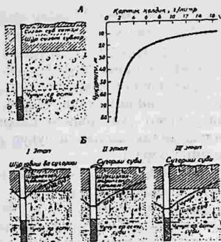
8.7.4.3-расм. Тик зовурнинг таъсир тизими: А-сув чиқариб олишдан олдин; Б-сув чиқариб олишдан кейин.
