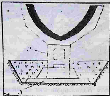
8.5.1.4-расм. Нов канал конструкция: 1-нов; 2-устун; 3-стакан типидagi пойдевор.
