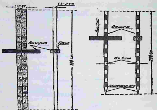
8.5.2.4-расм. Текислаш ишларини бажаришда қўлланиладиган рейка - визиркалар.
