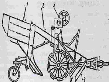
8.7.2.1-расм. КМ -800 мар- кали канаво- копатель 1 - ишчи орга- ни 2 - рамаси, 3 - кесиш ор- ганлари, 4-растегич
