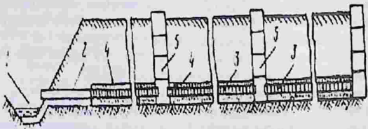
8.7.3.4-расм. Ёпиқ зовурнинг бўйлама қирқими:
