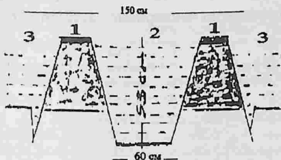
8.6.4.6-расм (а). Чек олгичнинг икки марта параллел ўтишидан ҳосил бўлган ўқариқ. 1-уват (марза); 2-ўқариқ; 3-чек.
