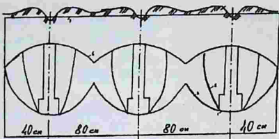
8.5.2.7-расм. Уч иш қуролига эга бўлган РУ-65-2,5 маркали чуқур юмшатгичнинг иш ҳолати.
