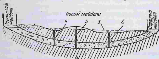
7.2-расм. Босимли сув ҳовузининг тузилиши.
