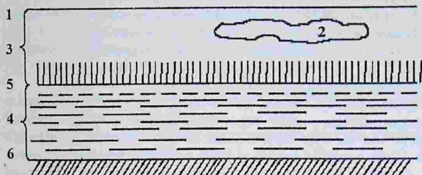
7.1-расм. Сизот ва тупроқ сувларининг жойлашиш тизими.
