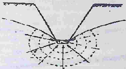
8.7.1.5-расм. Сизот сувнинг зовурга томон оқиб бериш тизими: 1-тенг босимли чизиқлар (эквипотенциаллар); 2-сув оқими чизиқлари.
