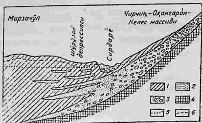
5.3.1-расм. Мирзачўл сизот сувларининг жойлашиш чуқурлиги ва гидрогеологик тизими.
