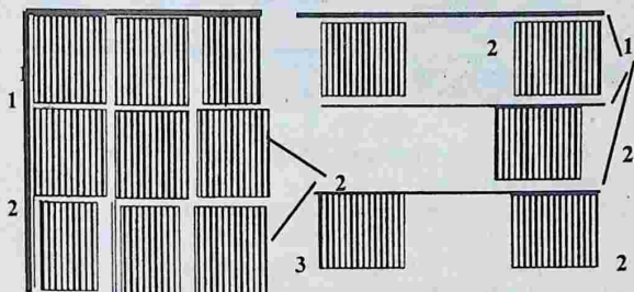
8.6.4.1-расм. Эгатлаб шўр ювишда бўйлама (а) ва кўндаланг (б) ўқариқларни жойлаштириш тизими.
