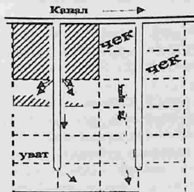
8.6.4.6-расм (а). Чек олгичнинг икки марта параллел ўтишидан ҳосил бўлган ўқариқ. 1-уват (марза); 2-ўқариқ; 3-чек.
