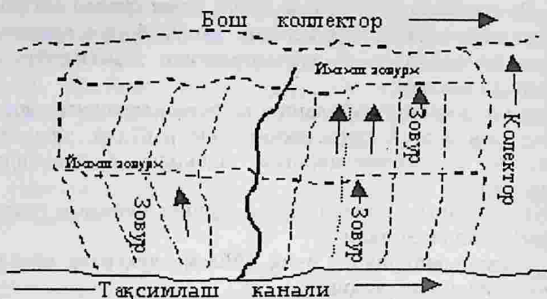
7.1.1-расм. Очиқ зовур ва коллекторлар тизими.
