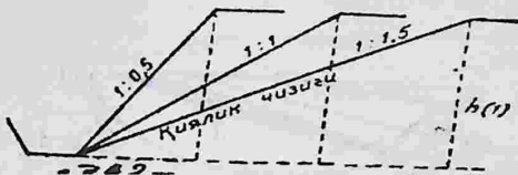
8.7.1.3-расм. Қиялик катталиги. h -зовур чуқурлиги.
