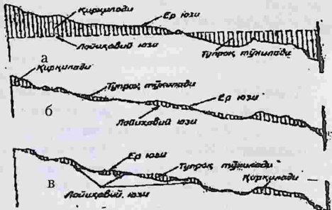
8.5.2.2-расм. Лўйиҳавий юзаларининг бўлиниши. А-ётиқ юза; б-қия юза; в-топографик юза.
