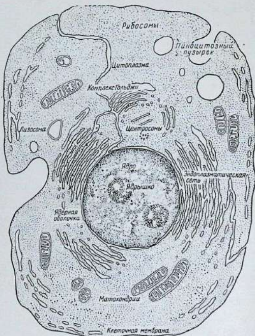
Рис. 2. Схема строения клетки под электронным микроскопом (по Браще, 1966).
