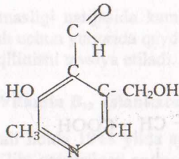
piridoksal
