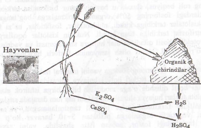
13- rasm. Olingugurtning tabiatda aylanishi.
