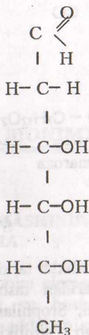
digitoksoza
