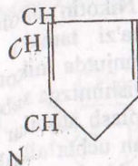
NH pirazol
