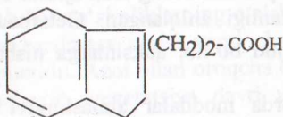
IMK
