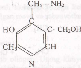
piridoksalamin
