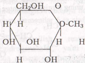
\nu -etilglikozid
