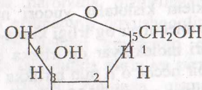
dezoksiriboza
