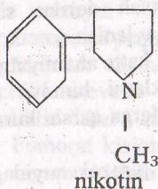
nikotin
