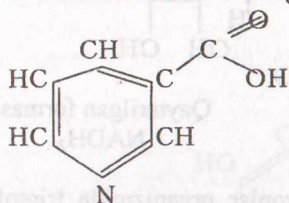
Nikotin kislota
