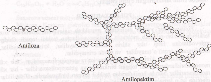
8-rasm. Amiloza va amilopektinning struktura tuzilishi
