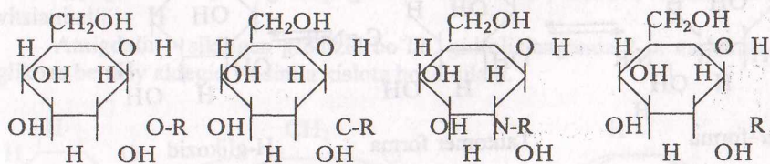
O - glikozid
