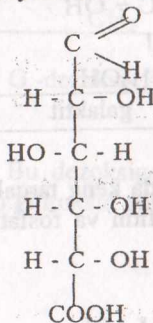
D-glyukuron kislota
