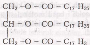
Triglitserid (prostearin)
