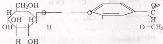
\alpha -forma
