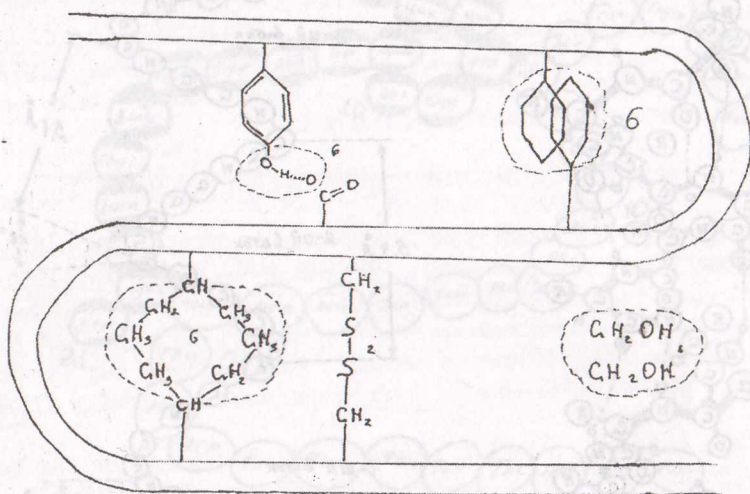
6-rasm. a- elektrostatik bog'lanish, b – vodorod bog'lari, v- qutbsiz yon zanjirlar bog'lanishi (yog' tomchisi),g- disulfid bog'lar, 2 ta qayramon chiziqli polipeptid zanjirni ko'rsatadi.
