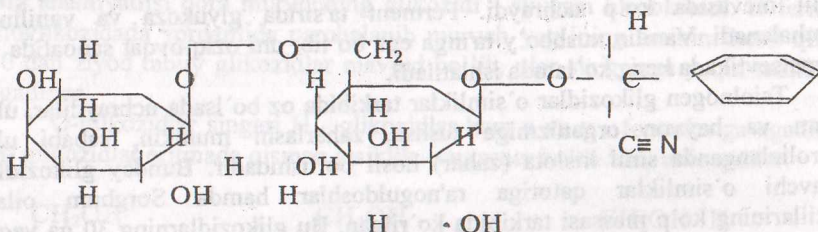
Vitsiatsin
