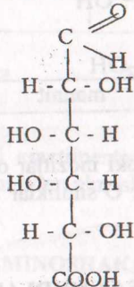
D-galakturon kislota
