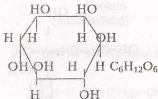
nozit
