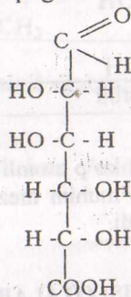
D-mankuron kislota
