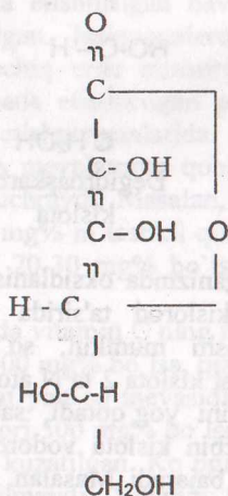
Askorbin kislota
