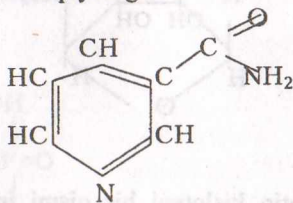
nikotinomid
