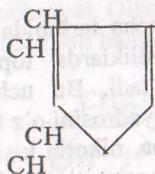
C tiofin
