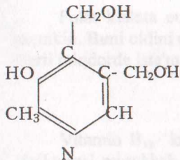
piridoksil
