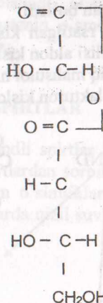
3-Ketoforma
