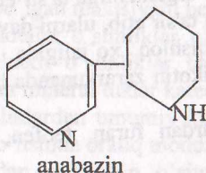
anabazin
