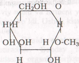
\alpha -etilglikozid
