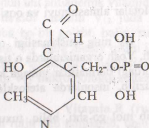
piridoksalfosfat
