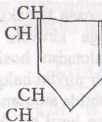
XH pirol
