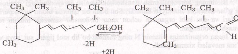
Retinol
