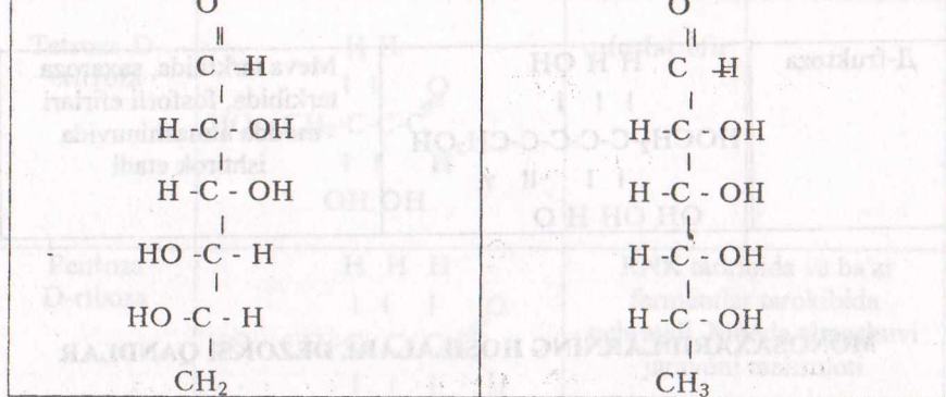
G-dezoksi-Z - mannoza
