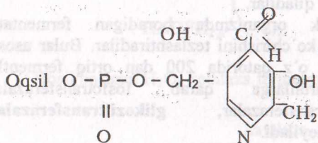
Piridoksalfement
