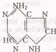
adenin
