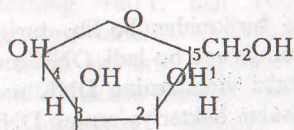
Riboza
