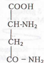
asparagin
