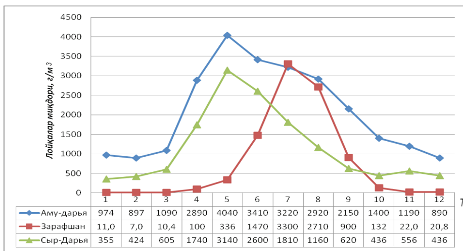
2-расм. Муаллақ ҳолда ҳаракатланувчи лойқалар миқдорининг вақтга нисбатан ўзгариши (Ўзбекистон ҳудудидан ўтувчи дарёлар).
