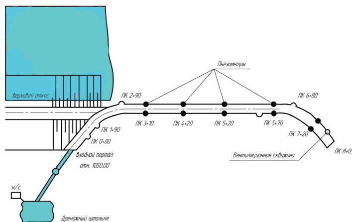
2-расм. Сизот сувлар ғоридаги пьезометр қувурлари жойлашув схемаси
