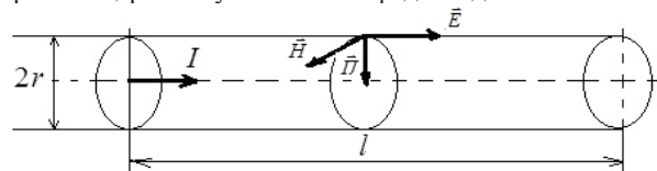
1-расм. Ўзгармас токли ўтказгичда энергиянинг ҳаракати.
