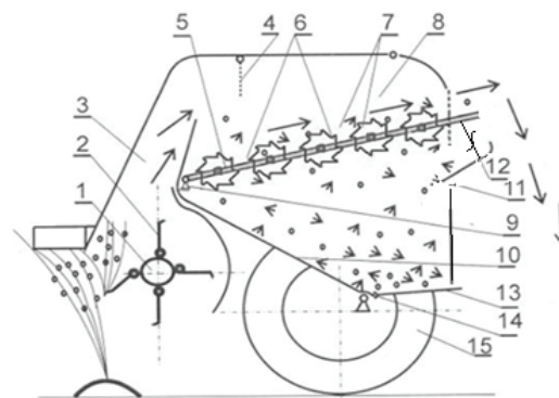
Расм. Чўл озукабоп ўсимликлари уруғ аралашмасини йиғувчи машинанинг технологик иш жараёни схемаси.
