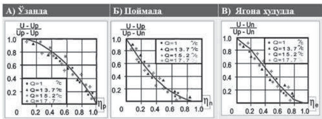
2-расм. Пойма ва ўзан оқимларнинг ўзаро таъсири зонасидаги тезликларнинг ўлчамсиз профиллари.
