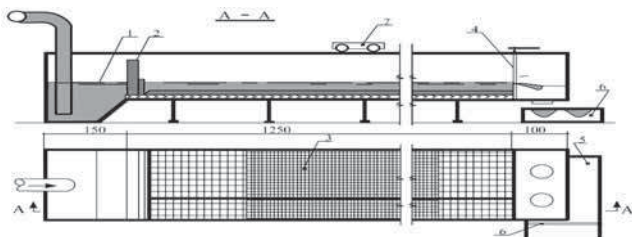
1-расм. Экспериментал лоток схемаси ва расми.
