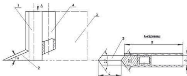
1-расм. Ғўза қатор ораларига кўп қаторлаб бугдой уруғини экувчи экикчининг тузилиши
