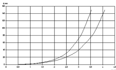
Рис.1. Допускаемые размывающие средние скорости потока для неоднородных несвязанных грунтов, при глубине размыва до 5% глубины наполнения канала и при коэффициенте однородности грунта, слагающего ложе канала K_0=0,5 , V_p , м/с.
