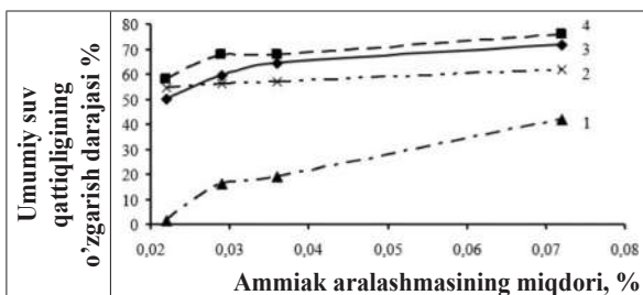
4-rasm. Ammiakning suvli eritmasi kontsentratsiyasi-ga qarab suvning umumiy qattiqligining o'zgarish darajasi 15°C va 40°C suv haroratida: 1-15°C da aralashmasdan yerosti qattiq suvi; 2-36 soatdan keyin 15°C da aralashtirmasdan yerosti qattiq suvi; 3-15°C da aralashtirilgandan keyin yerosti qattiq suvi; 4-40°C da aralashtirgandan keyin yerosti qattiq suvi.
