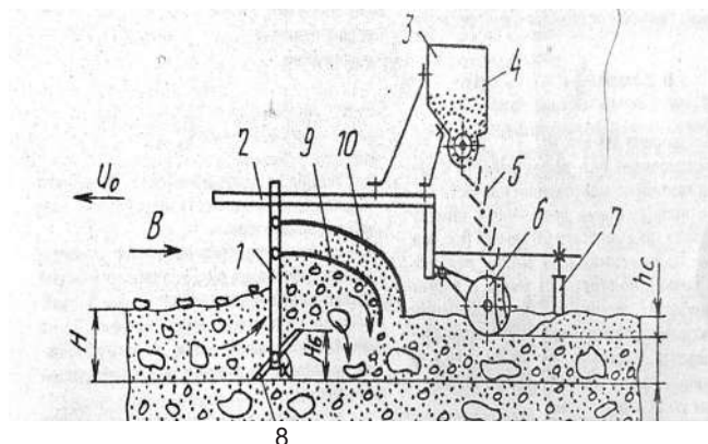
Рис 1. Устройство для заделки семян в каменистую почву.
