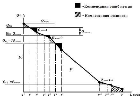
1-расм. Реактив қувватнинг кўп поғонали ўзгариш юкларининг ҳолати.
