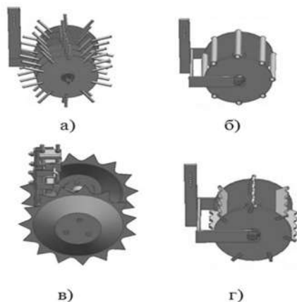
а – игнасимон; б – қувурсимон; в – диски-тишли; г – планкасимон
