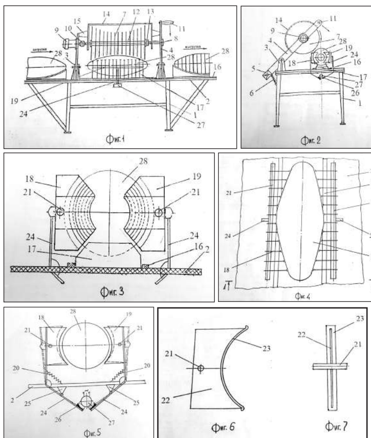
Рис. 1. Устройство для разрезания очищенного плода дыне на кольцевые дольки.
