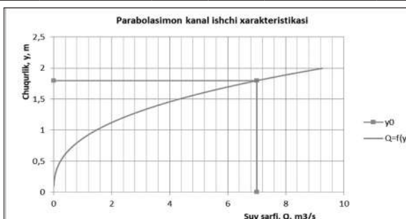
3-rasm. Parabola shaklidagi kanalning ishchi xarakteristikasi.
