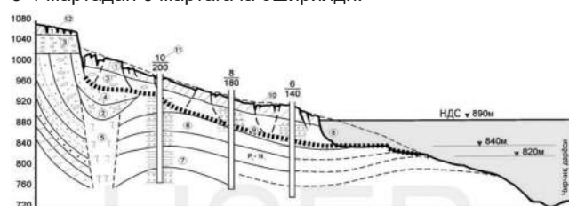
1.1-расм. Мингчукур кўчкисининг геологик профили.
