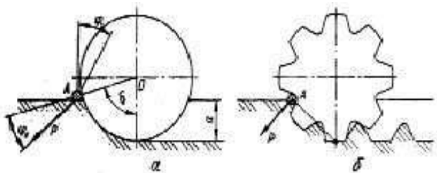
5-rasm. Borona diskklari. a-sferik disk b-kesik disk.
