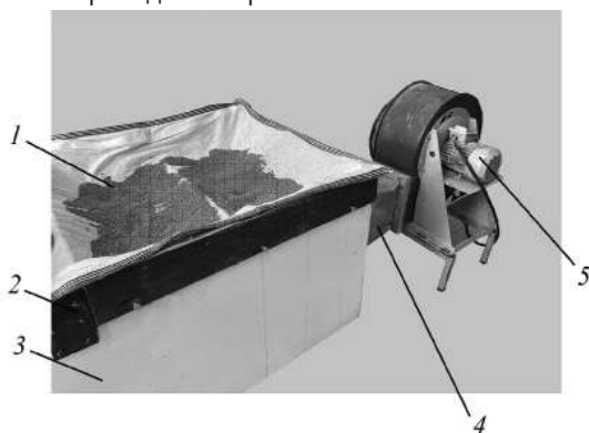
2-расм. Кўрт уруғини қуритувчи ускунанинг умумий кўриниши:
