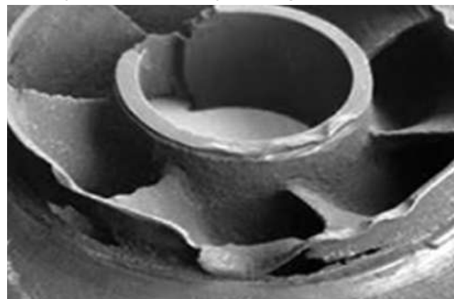
Ishchi g'ildirak kavitatsiya tasirida yemirilishi.
