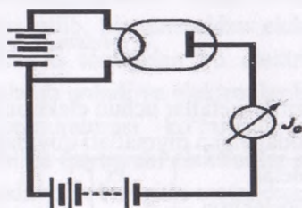
8.3-rasm. Vaakuumli diod lampasi
