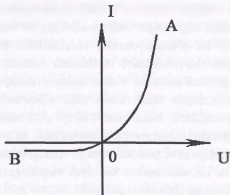
8.21-rasm. Diodda tokning kuchlanishga bog'liqlik grafigi
