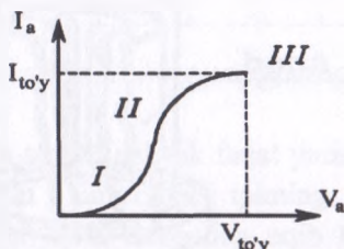
8.5-rasm. Anod tokining anod kuchlanishga bog‘liqlik grafigi
