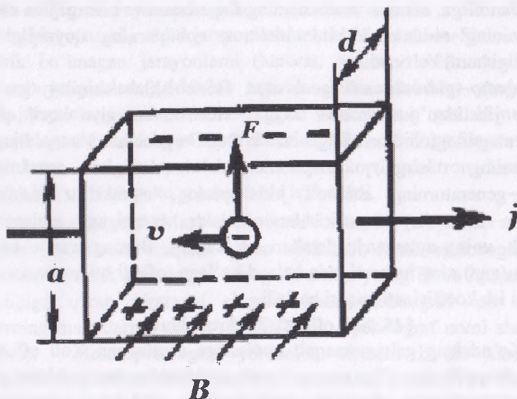
10.4-rasm. Xoll effektini aniqlash chizmasi
