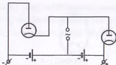
8.8-rasm. Ikki yarim davrli to'g'rilagich sxemasi
