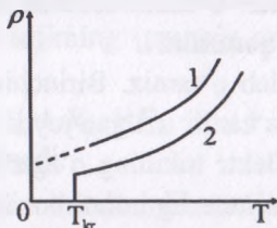
5.6-rasm. Solishtirma qarshilikning haroratdan bog'liqligi
