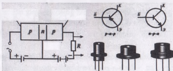
8.25. Tranzistorlarning ko'rinishi va ulanishi
