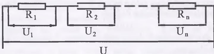
5.4-rasm. O‘tkazgichlarni ketma-ket ulash
