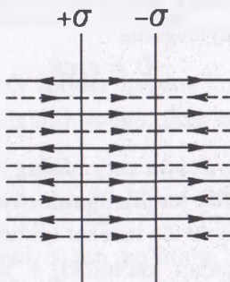
2.3-rasm. Zaryadlangan parallel tekisliklar maydoni
