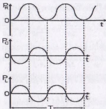
14.11-rasm. Quvvatlarning vaqtga bog'liqlik grafiklari
