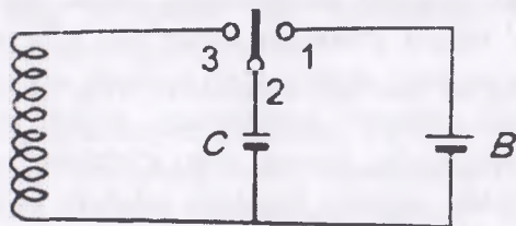
14.1-rasm. Elektr tebranish konturi
