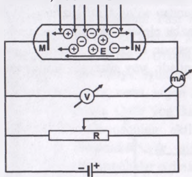
7.1-rasm. Gazlarda elektr tokini aniqlash qurilmasi
