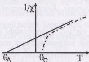
13.16-rasm. Ferritlarning magnit qabul qiluvchanligining temperaturaga bog'liqligi
