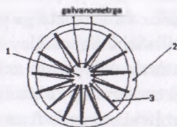
8.27-rasm. Aktinometr termobatareyasi
