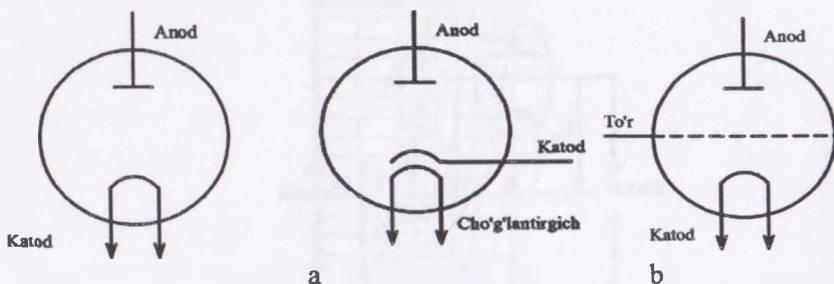
8.14—rasm. Vakuimli elektron lampalar
