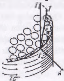
13.3-rasm. Mikroskopik yupqa sirt yaqinidagi qatlamda magnitlanish vektori
