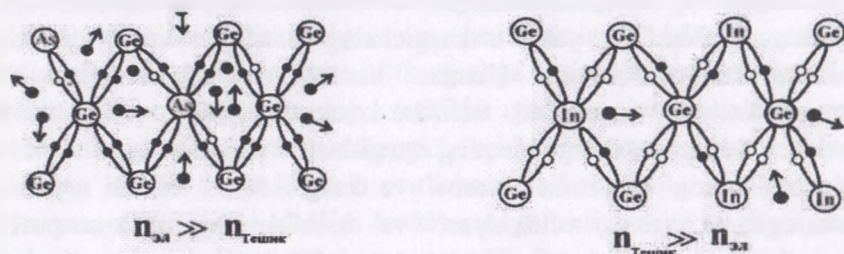
8.22 rasm. Germaniy atomlari orasidagi elektron bog'lanishlar joylashgan .
