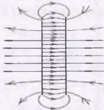
4.6-rasm. Yassi kondensatorda kuch chiziqlari
