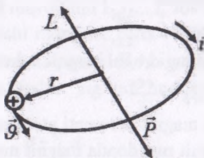
13.7-rasm. Elektronlarning orbital harakati
