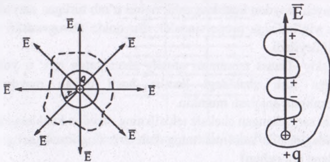
2.1–rasm. Nuqtaviy zaryad va jismning maydoni
