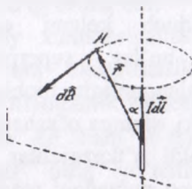
9.4-rasm. Tok elementi magnit induktsiyasini hisoblash chizmasi
