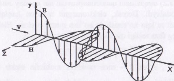
15.1—rasmda. Yassi elektromagnit to'loinning biror vaqt lahzasidagi fotosurati
