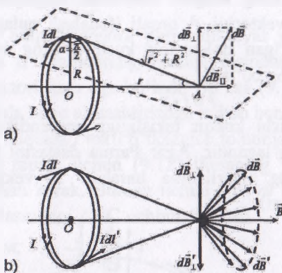
9.8 -rasm. Aylanma tok maydonini hisoblash chizmasi
