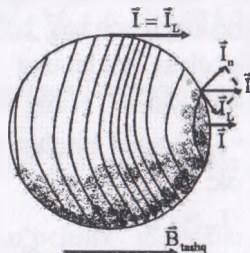
13.4-rasm. Sirt molekulyar toklarining bir jinsli magnitlangan sharti
