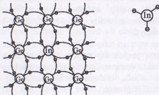
8.18-rasm. P-tip yarimo'tkazuvchanlik hosil qilish
