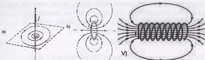
9.3 – rasm. Magnit induksiya chiziqlari
