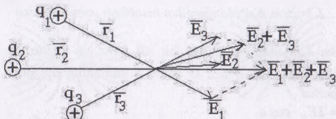
1.4-rasm. Superpozitsiya prinsipini namayon qiluvchi chizma
