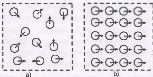
13.1 – rasm. Magnit momentlari maydon bo'ylab orientirlanishi
