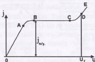
7.3-rasm. Mustaqil gaz razryadi volt-ampere xarakteristikasi
