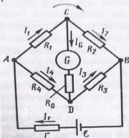
14.8-rasm. Uitsonning noma'lum qarshilikni o'lchash qurilmasi
