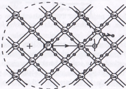
8.16—rasm. Aralashmali yarimo'tkazgich hosil qilish
