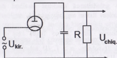
8.7-rasm. Bir yarim davrli to'g'rilagich sxemasi
