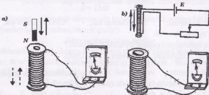
12.1-rasm. Elektronmagnit induksiya hodissini kuzatish
