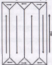
13.14-rasm. Domenlarning magnit momentlari
