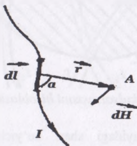
11.4.-rasm. Bio-Savar-Laplaslar qonunini hisoblash chizmasi
