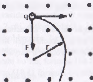
10.2-rasm. Harakatlanayotgan zarraga ta'sir qiluvchi kuchni aniqlash
