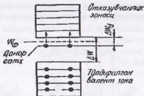
8.17-rasm. Yarimo'tkazgichlarda zonalarining joylashuvi
