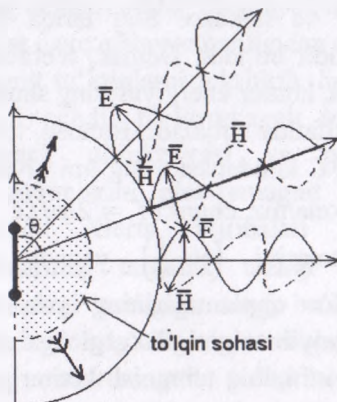
15.3-rasm. Nurlagichdan tarqalayotgan to'qlinlar
