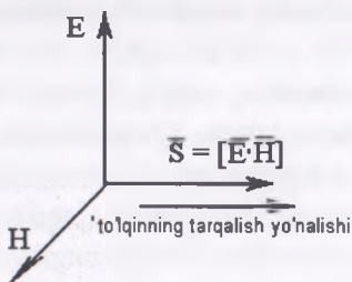
15.6-rasm. S , E , H vektorlarning o'zaro perpendikulyarligi
