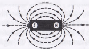
9.2- rasm. Magnit sterjening magnit induksiya chiziqlari.
