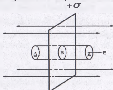
2.2-rasm. Zaryadlangan tekislik maydoni
