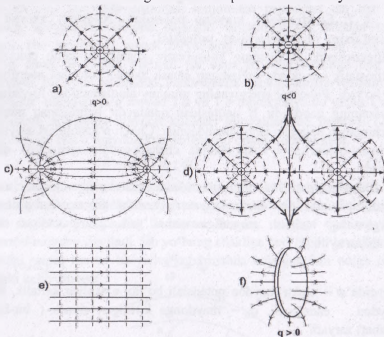
2.6-rasm. Ekvipotensial sirtlar ko'rinishlari
