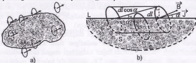
13.2-rasm. To'la molekulyar tokni topish chizmasi
