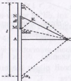
9.6-rasm. O'tkazgichning elementar qismi dl tomonidan hosil qilingan magnit induksiya
