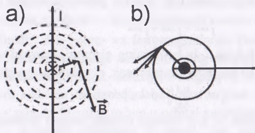
13.6-rasm. O'tkazgichning magnit maydonini
