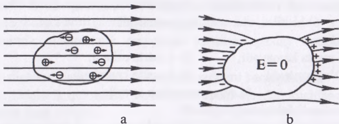
4.1-a'b rasm. O'tkazgichlar elektr maydonida
