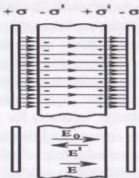
3.2-rasm. Dielektrikning qutblanish jarayoni
