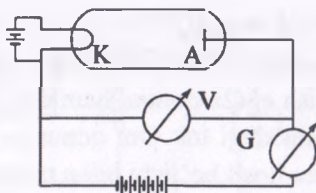
8.4-rasm. Termoelektron hodisani tajribada qurilmasi
