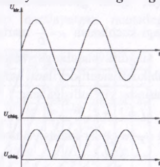
8.9-rasm. Kuchlanishning vaqtga bog'liqlik grafigi
