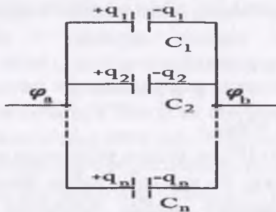
4.4-rasm. Kondensatorlarni parallel ulash
