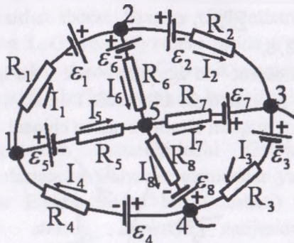
5.13-rasm. Umumiy ko‘rinishdagi tarmoqlangan zanjir
