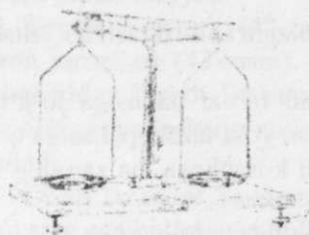
43-rasm. Texnik kimyoviy tarozi va uning toshlari: 1-kolonka; 2-arreir; 3-tarozi-ning pallalari; 4-strelka; 5-shkala; 6-shovun; 7-tarozi gorizontal holatni to'g'rilash uchun vint; 8-velka; 9-tarozi pallasini to'g'rilash uchun vint.
