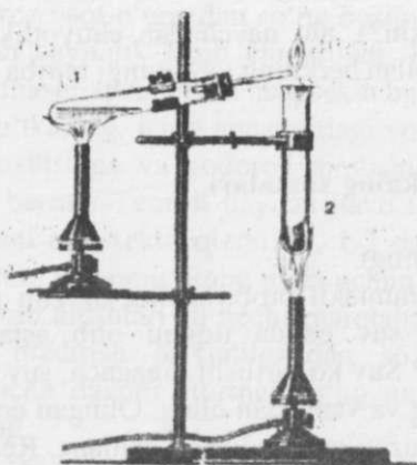
76-rasm. Ammiakni kislorodda yondirish uchun asbob:
