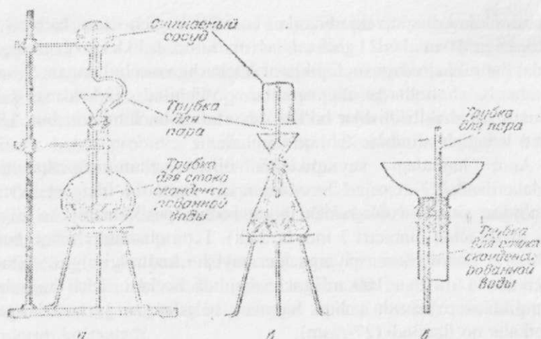
29- rasm. Idishlarni par bilan yuvuvchi asbob
