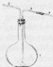
51-rasm. Yuvgich: 1-tagi yassi kolba; 2-o'tmas burchak ostida egilgan trubka; 3-o'tkir burchak ostida egilgan trubka; 4-uchi cho'zilean trubka.
