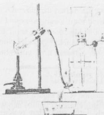
Gazometrni kislorod gazi bilan to'ldirish: 1 va 2 jo'iraklar, 3-voronka; 4-tubus.
