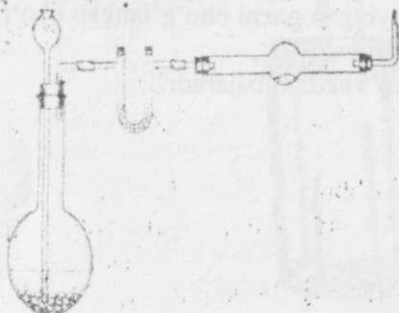
68-rasm. Vodorodning qaytaruvchilik xossalarini o'rganish uchun asbob
