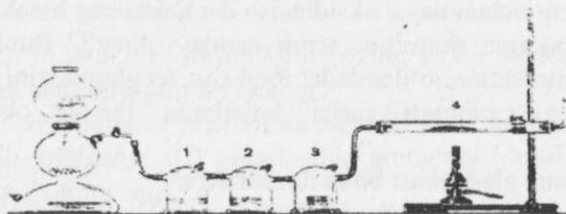
84-rasm. Qaytarilgan temirni olinishi: 1,2,3.-yuvuchi Tishenko idishlari; 4-o'tga chidamli shisha naycha
