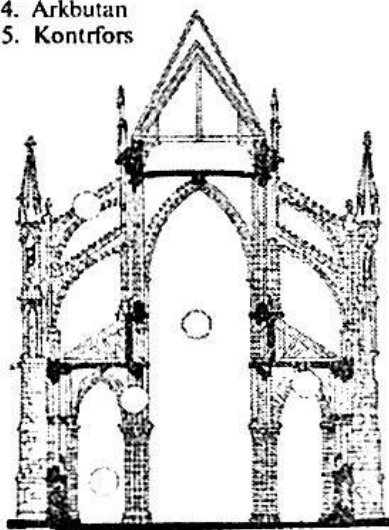
11-rasm. Roman va gotika konstruktiv xususiyatlari
