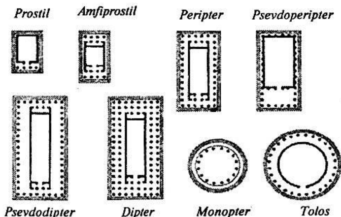
24-rasm. Ibodatxona turlari. Qadimgi Yunoniston
