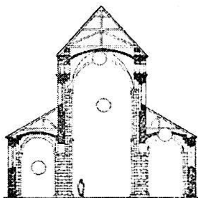
11-rasm. Roman va gotika konstruktiv xususiyatlari
