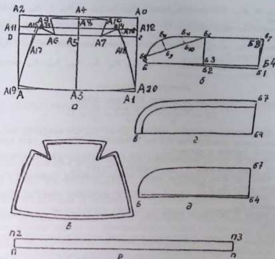
Рис. 50. Построение мужской цельношерстной шапки типа «москвичка» а—головка; б—бортик из меха; в—подбортик; г—подборка
