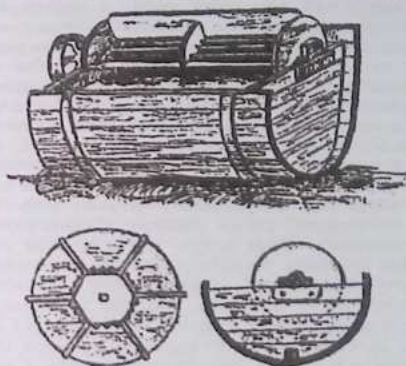
Рис. 23. Устройство гашпиля
