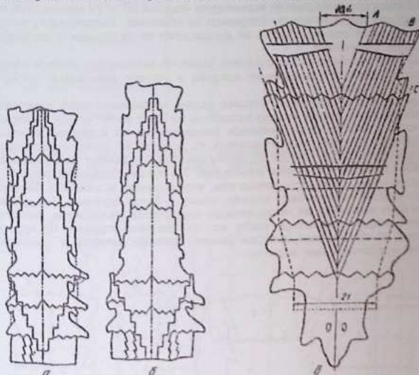
Рис. 41. Шкурки каракуля до (а) и после (б) ступенчатого раскроя и V-образногоrostука (в)
