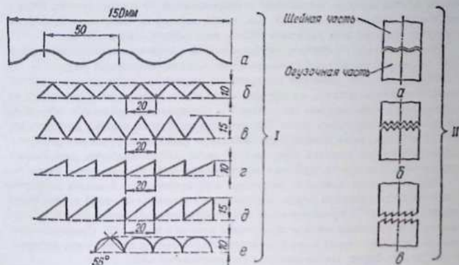
Рис.135. Соединительные пилки (I) и соединение шкурок при помощи пилок (II)
