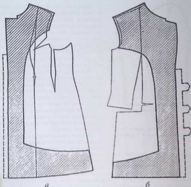
Рис.131. Расположение и формы каркасных прокладок: а — для женской одежды; б — для мужской одежды
