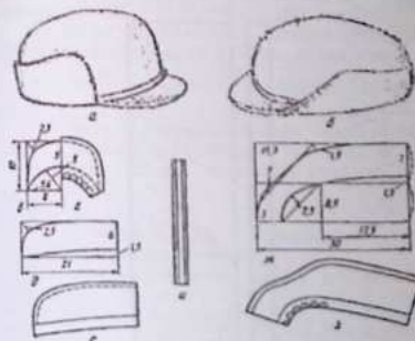
Рис. 48. Шапки с козырьком (а) и окол, переходящим в козырек (б); формы для раскройки козырька (в, д), лицевых и подлицевых наушников (е, ж), наушников с подкозырьком (ж, з)
