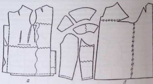
Рис. 38. Соединение оцки при изготовлении пальто: а—волнистое и пилообразное; б—косая пилка.
