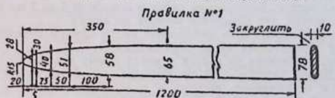
Рис. 5. Чертеж прави́лки для шкурок голубого песка.
