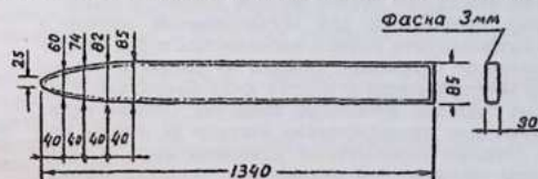
Рис. 5. Чертеж прави́лки для шкурок голубого песка.
