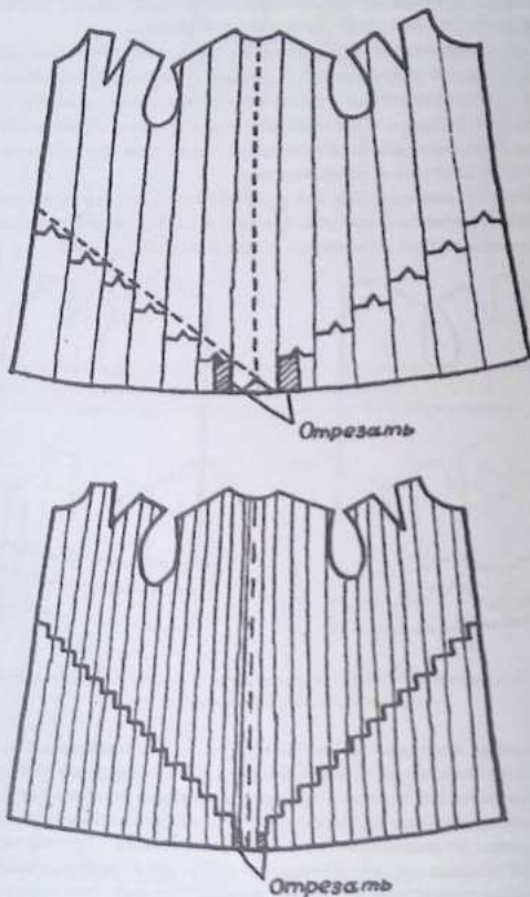
Рис. 141. Схема ступенчатой перерезки полос с перемещением для удлинения стана
