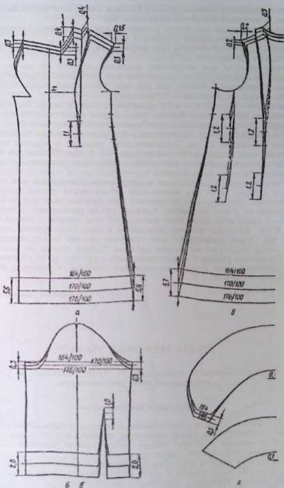
Рис. 36. Изменение размеров лесал деталей скроя при изменении роста изделия.
