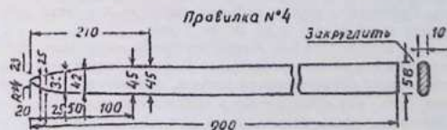
Рис. 6. Чертежи прави́лок для шкурок норки.
