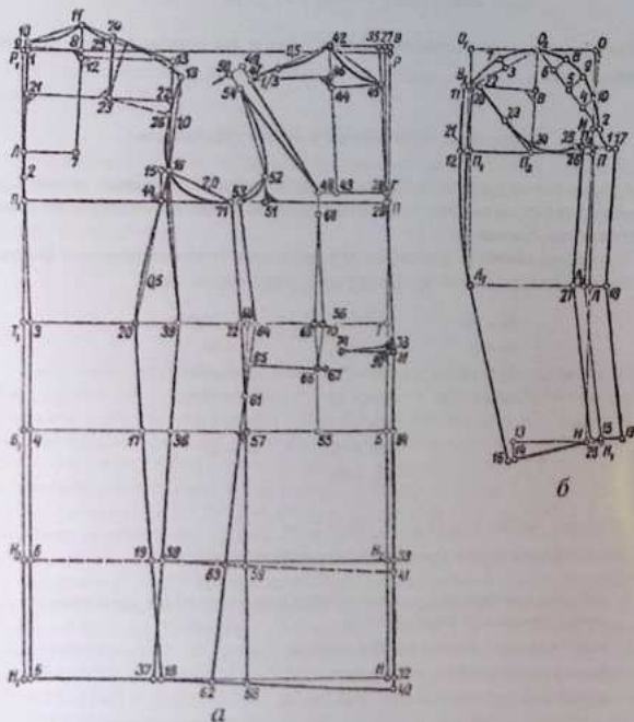
Рис. 120. Построение чертежа основы второго варианта пиджа (полушубто) мужского: а — спинка, полочка и бочок; б — рукав
