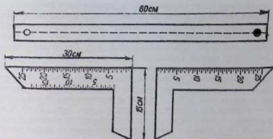
Рис.114. Специальная линейка и угольник для измерения проекционных величин
