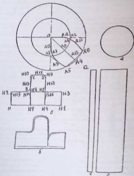
Рис. 49. Построение мужской шапки ушанки: а—клины; б—назатыльник, наушник, козырек, в—назатыльник, наушник и козырек из меха; г—дольник; д—основание; е—подборка
