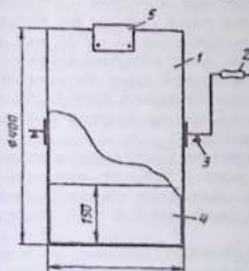
Рис. 27. Барабан для выделки кожи 1 — корпус, 2 — привод ручной или через электрический редуктор, 3 — подпирник, 4 — лопасть, 5 — крышка люка.
