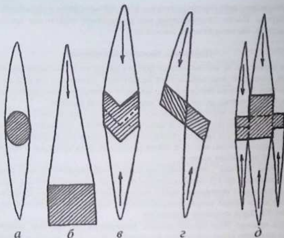
Рис. 138. Способы удаления пороков мехового верха изделия: а — прорезка "рыбкой"; б — спуск клина; в — спуск клинцев с двух сторон; г — спуск клинцев параллельный; д — многоклинный спуск. Штриховкой отмечены удаляемые участки с повреждениями
