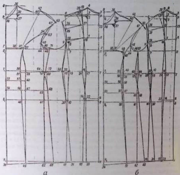
Рис. 122. Построение чертежей основ женского пажа: а — для фигур второго типа; б — для фигур третьего типа
