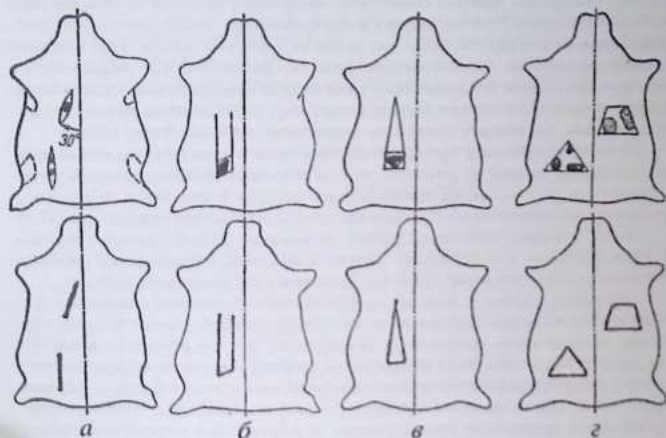
Рис.133. Способы удаления дефектов: а — прорезка «рыбкой»; б — вытяжка; в — спуск клина; г — вставка
