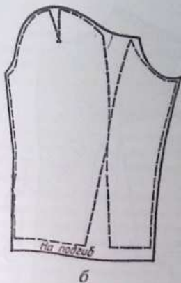
Рис. 130. Оформление лекал меховых скроев (а — станы, б — рукава)
