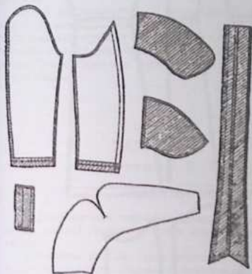
Рис. 42. Лекала деталей женского пальто из велюродоподобного материала
