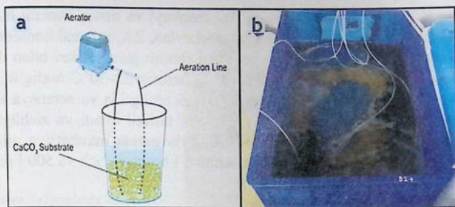
3-rasm. (a) Nitrikatsiyalovchi bakteriyalar reaktorining sxematik diagrammasi [11, 13]; (b) nitrikatsiyalovchi bakteriyalarning haqiqiy kulturasi
