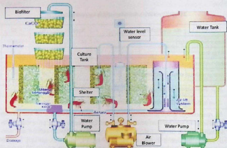
7-rasm. Vertikal xomashyo boshpanalaridan foydalanigan holda o'stirish bosqichida krevetkarni yetishtirish sxemasi [1]
