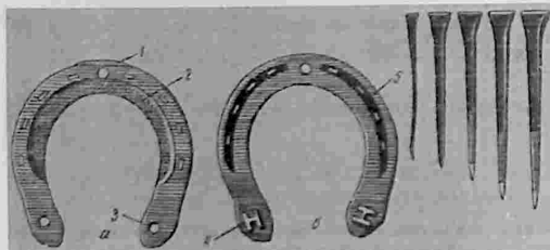
Tishlari almashinadigan orqa oyoq taqasi: Taqa mixlari. (107-rasm)
