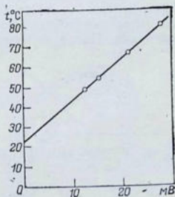
Рис. 8.15. Градуировочный график термопары.
