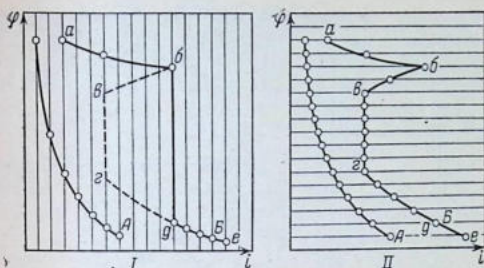
Рис. 14.8. Диаграммы, поясняющие гальваностатический (I) и потенциостатический (II) методы снятия поляризационных кривых.
