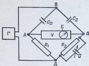
Рис. 3.8. Принципиальная схема прибора Е8-1.
