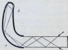
Рис. 4.17. Схема кюветы (прямые возбуждающие лучи отводятся в загнутую часть и поглощаются).
