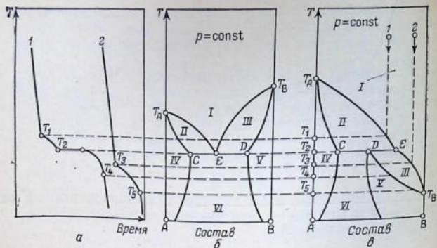
Рис. 8.13. Кривые охлаждения (а) и диаграммы плавкости (б) и (в) систем с ограниченной растворимостью компонентов в твердом состоянии.
