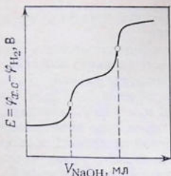
Рис. 13.20. Вид кривой титрования хромовой кислоты едким натром.
