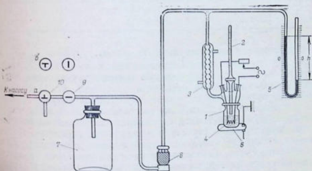
Рис. 7.1. Схема установки для определения давления насыщенного пара легколетучих жидкостей:
