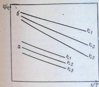
Рис. 14.5. Зависимость \lg i_\eta от 1/T :
