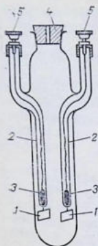
Рис. 11.4. Сосуд для определения сопротивления: 1 — платинированные платиновые электроды; 2 — стеклянные трубки; 3 — легкоплавкий сплав; 4 — пробка; 5 — клеммы.
