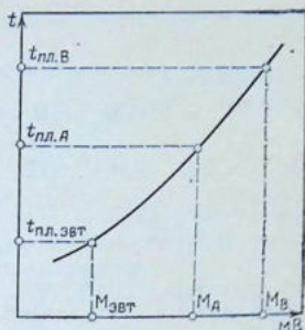
Рис. 8.17. Градуировочный график термомпары.
