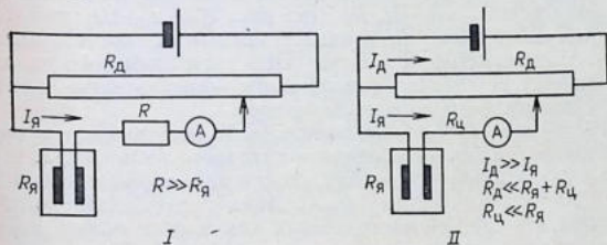
Рис. 14.9. Принципиальные схемы цепей поляризации гальваностатического (I) и потенциостатического (II) методов:
