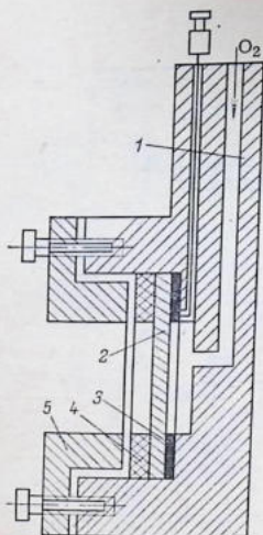
Рис. 13.8. Кислородный электрод:
