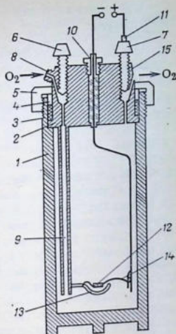
Рис. 5.6. Схема калориметра для определения теплот сгорания:
