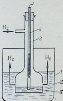
Рис. 13.21. Водородный электрод для потенциометрического титрования:
