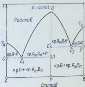
Рис. 8.11. Диаграмма плавкости не-изоморфной смеси, образующей устойчивое химическое соединение.
