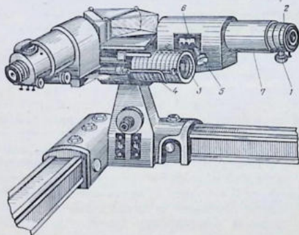
Рис. 4.22. Внешний вид универсального монохроматора УМ-2:
