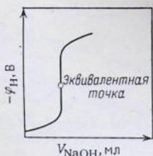
Рис. 13.16. Вид кривой титрования хлороводородной кислоты едким натром.
