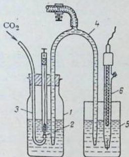
Рис. 13.10. Схема гальванического элемента с окислительно-восстановительным электродом:
