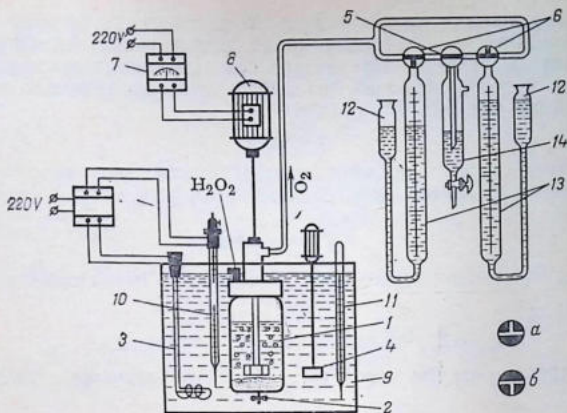
Рис. 10.6. Схема установки для изучения кинетики гетерогеннокаталитического разложения пероксида водорода:
