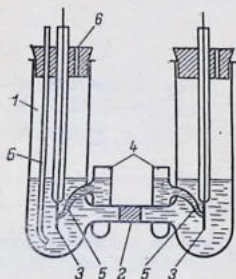
Рис. 14.17. Электрохимическая ячейка для изучения поляризации гальванического элемента:
