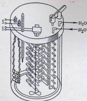
Рис. 8.8. Прибор для изучения взаимной растворимости двух жидкостей.
