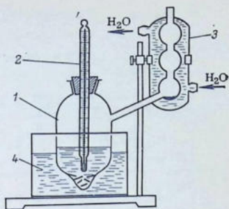
Рис. 8.6. Прибор для определения температур кипения жидких смесей:
