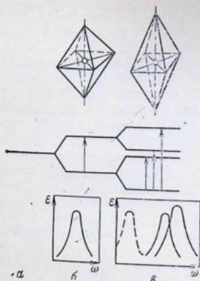
Рис. 4.31. Схема расщепления термина иона \text{Cu}^{2+} в поле молекул адденда и происхождения полосы поглощения:
