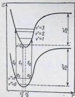
Рис. 4.7. Переходы с поглощением энергии между двумя электронными состояниями двухатомной молекулы. Иллюстрация принципа Франка — Кондона:
