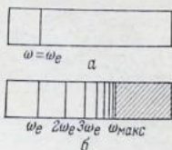
Рис. 4.4. Схема спектров гармонического (а) и ангармонического (б) осцилляторов.
