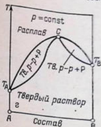
Рис. 8.14. Кривые охлаждения и диаграммы фаз (г) изоморфных систем.
