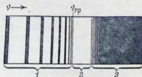
Рис. 4.20. Общий вид спектра поглощения:
