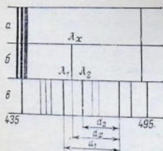
Рис. 4.18. Расшифровка спектров комбинационного рассеяния:
