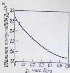
Рис. 3.11. График функции p_2 = \varphi(g_2) для раствора ацетона в бензоле.
