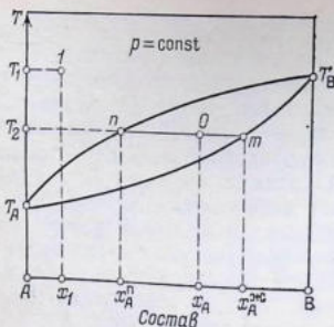
Рис. 8.5. Диаграмма кипения системы без азеотропной смеси.
