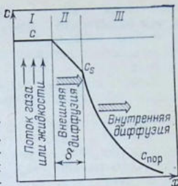
Рис. 10.1. Распределение концентрации реагирующего вещества у поверхности и внутри зерна катализатора:
