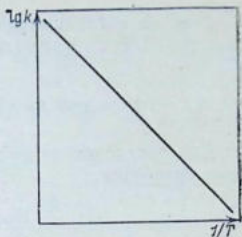
Рис. 9.2. Зависимость логарифма константы скорости реакции от обратной температуры.
