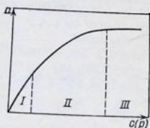
Рис. 10.2. Изотерма адсорбции по Лэнгмюру.
