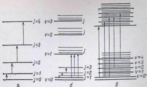
Рис. 4.1. Энергетические уровни молекул и переходы:
