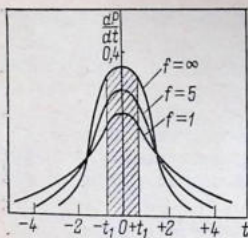
Рис. 1.2. График функции распределения Стьюдента для различных чисел степеней свободы f .
