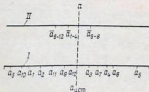
Рис. 1.1. Распределение результатов отдельных измерений (I) и выборочных значений средних арифметических (II) относительно истинного значения величины a .
