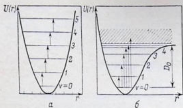
Рис. 4.3. Энергетические уровни и переходы между ними для гармонического осциллятора (а) и реальной молекулы (б).
