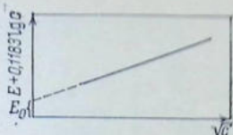
Рис. 13.15. Вид графика при определении коэффициента активности раствора хлороводородной кислоты.
