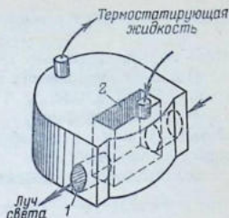
Рис. 4.30. Приспособление для термостатирования кюветы в фотоэлектроколориметрах ФЭК-М и ФЭКН-57:
