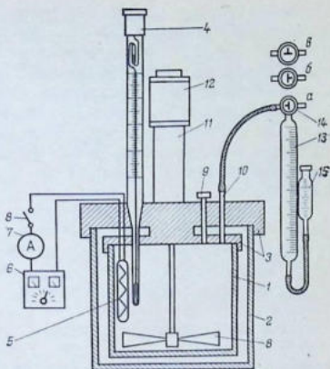
Рис. 5.5. Схема калориметра для определения теплот гетерогенно-каталитических реакций гидрирования в жидкой фазе:
