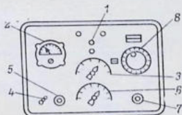
Рис. 3.9. Внешняя панель прибора Е8-1:
