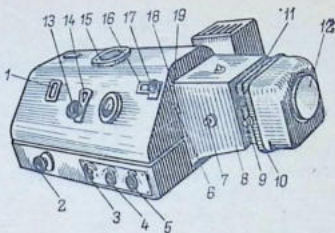
Рис. 4.25. Спектрофотометр СФ-4:
