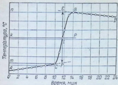
Рис. 5.4. Изменение температуры во время калориметрического опыта.
