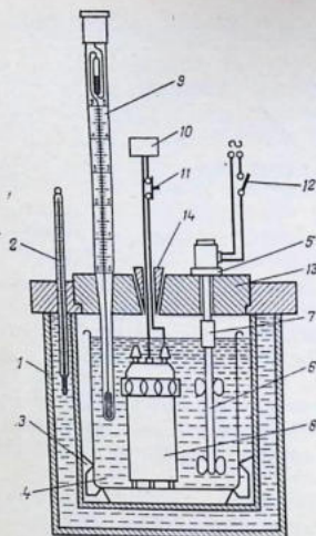
Рис. 5.6. Схема калориметра для определения теплот сгорания:
