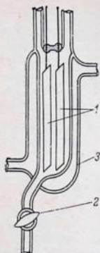
Рис. 3.10. Измерительный конденсатор:
