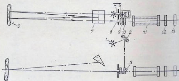
Рис. 4.24. Оптическая схема спектрофотометра СФ-4:
