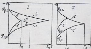
Рис. 14.15. Поляризационные диаграммы гальванических элементов:
