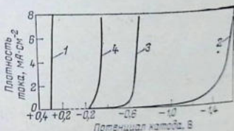
Рис. 14.3. Поляризация при катодном осаждении некоторых металлов:
