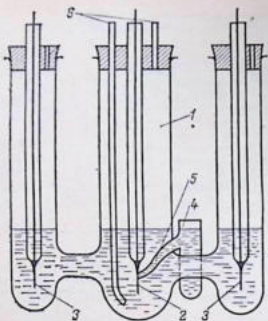
Рис. 14.10. Электрохимическая ячейка: 1 — стеклянный сосуд; 2 — рабочий электрод; 3 — вспомогательные электроды; 4 — промежуточный сосуд; 5 — электролитический ключ с капиллярным концом; 6 — трубки для входа и выхода газа.
