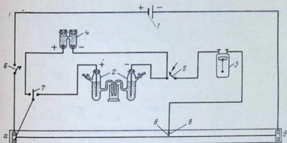
Рис. 13.2. Схема установки для определения э.д.с. компенсационным методом:
