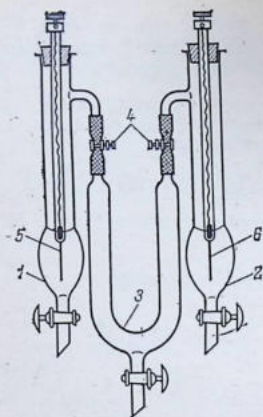
Рис. 12.2. Электролизер для определения чисел переноса ионов:
