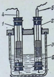
Рис. 13.5. Схема гальванического элемента Якоби — Даниэля:
