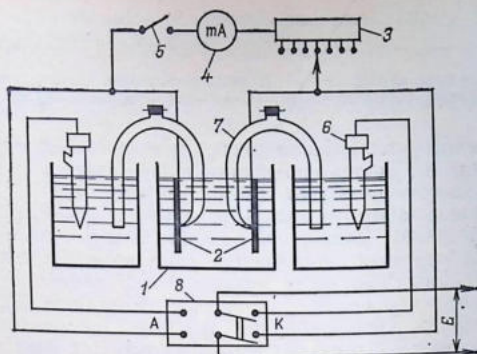
Рис. 14.16. Схема установки для изучения поляризации гальванического элемента:
