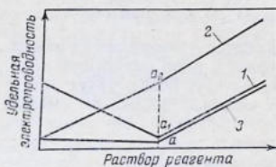
Рис. 11.6. Вид кривых при кондуктометрическом титровании:
