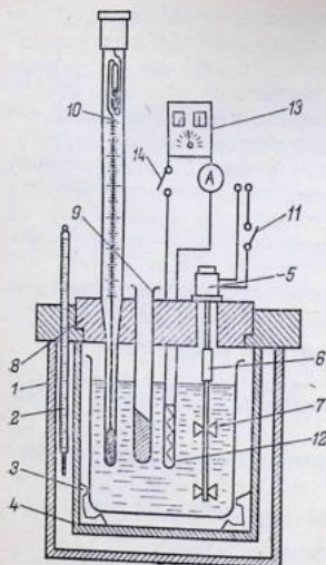
Рис. 5.1. Схема калориметра с изотермической оболочкой:
