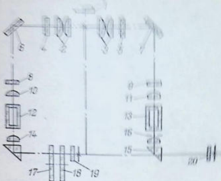
Рис. 4.26. Оптическая схема фотоэлектроколориметра ФЭК-М:
