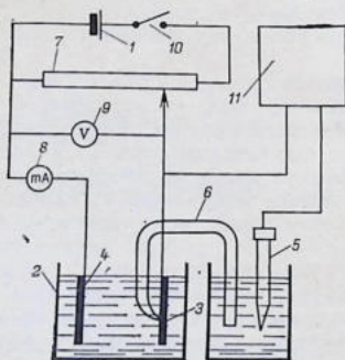
Рис. 14.7. Принципиальная схема установки для измерения электродных потенциалов под током:
