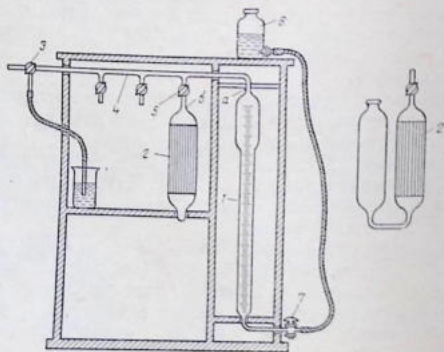
Рис. 6.2. Схема газоанализатора (аппарат Орса):
