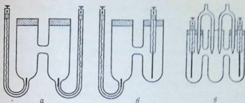
Рис. 13.6. Стекланные сосуды для потенциметрических измерений в термостате.
