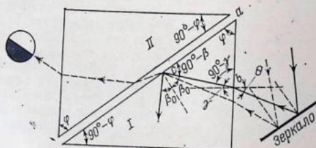
Рис. 3.3. Схема хода лучей в призмах рефрактометра типа Аббе.
