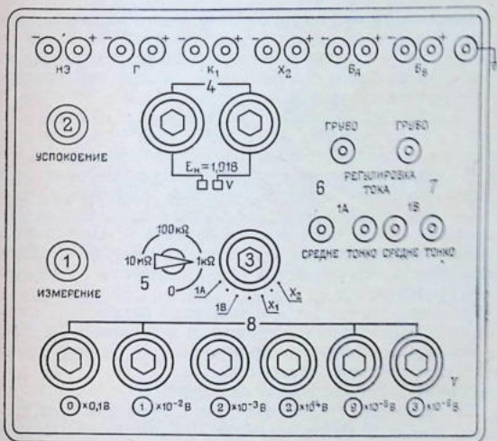
Рис. 13.4. Внешняя панель потенциометра РЗ7-1:
