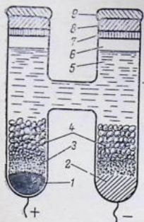
Рис. 13.3. Нормальный элемент Вестона: 1 — ртуть; 2 — амальгама кадмия; 3 — смесь \text{CdSO}_4 \cdot \frac{8}{3}\text{H}_2\text{O} и \text{Hg}_2\text{SO}_4 ; 4 — кристаллы \text{CdSO}_4 \cdot \frac{8}{3}\text{H}_2\text{O} ; 5 — насыщенный раствор \text{CdSO}_4 ; 6 — воздушный пузырек; 7 — парафин; 8 — пробка; 9 — менделеевская замазка.
