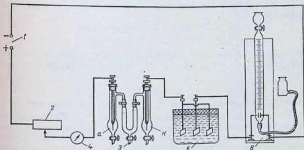
Рис. 12.1. Схема установки для определения чисел переноса ионов:
