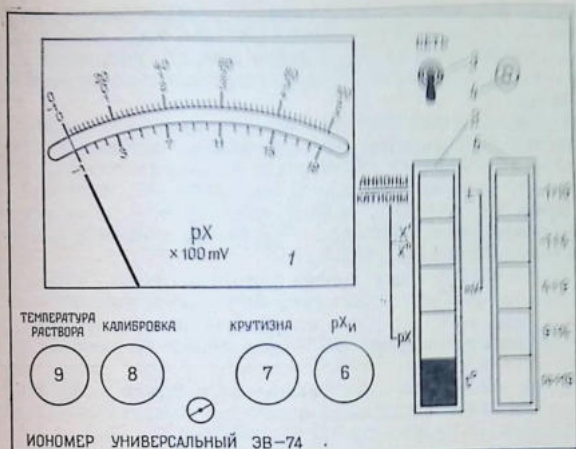
Рис. 13.14. Внешняя панель иономера ЭВ-74.
