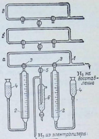
Рис. 10.5. Система бюреток для измерения скорости поглощения водорода:
