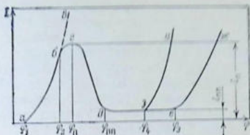
Рис. 14.4. Анодная потенциостатическая поляризационная кривая для металла, способного пассивироваться (см. пояснения в тексте).
