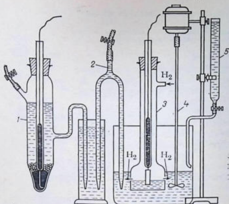
Рис. 13.22. Схема гальванической цепи при потенциметрическом титровании: 1 — каломельный электрод; 2 — солевой мостик; 3 — водородный электрод; 4 — мешалка; 5 — бюретка.
