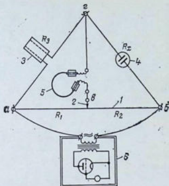
Рис. 11.2. Схема установки для определения электропроводности:
