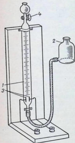
Рис. 12.4. Газовый кулонометр:
