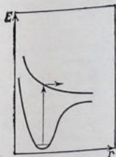
Рис. 4.8. Переходы с поглощением энергии между основным и первым возбужденным состоянием молекулы \Gamma_2 . Иллюстрация принципа Франка — Кондона:
