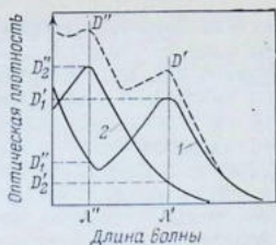
Рис. 4.11. Полоса поглощения, имеющая форму кривой Гаусса.
