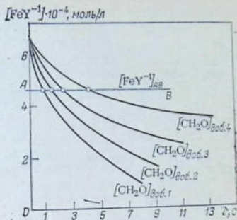
Рис. 9.4. Кинетические кривые восстановления \text{FeY}^{-1} в зависимости от концентрации добавки формальдегида [\text{CH}_2\text{O}]_{\text{доб.}} .
