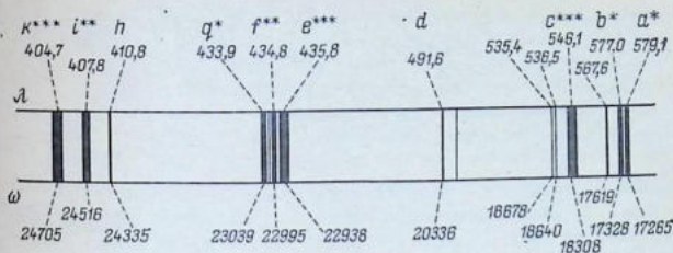
Рис. 4.14. Схема расположения линий в спектре ртути.
