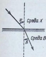
Рис. 3.1. Преломление луча на границе двух прозрачных сред.
