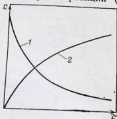
Рис. 9.1. Изменение концентрации c одного из исходных веществ 1 и одного из продуктов реакции 2 при протекании химической реакции.
