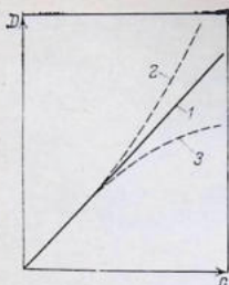
Рис. 4.10. Зависимость оптической плотности от концентрации раствора:
