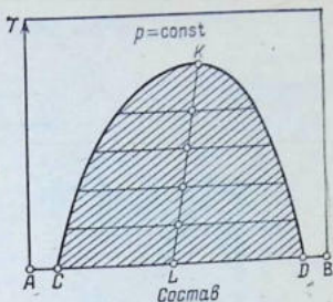
Рис. 8.7. Диаграмма растворимости для ограниченно смешивающихся жидкостей с верхней критической температурой растворения.
