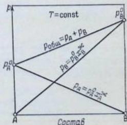
Рис. 8.1. Изотерма зависимости общего и парциальных давлений пара от состава идеального раствора.
