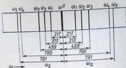
Рис. 4.6. Схема спектра комбинационного рассеяния \text{CCl}_4 .
