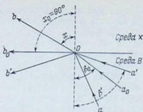
Рис. 3.1. Преломление луча на границе двух прозрачных сред.
