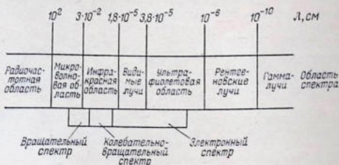
Рис. 4.2. Схема электромагнитного спектра.
