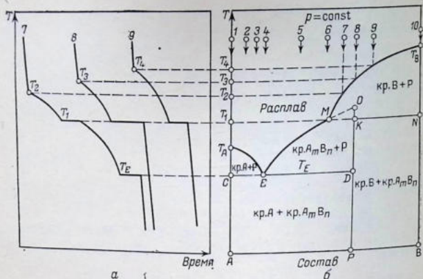
Рис. 8.12. Кривые охлаждения (а) и диаграмма плавкости (б) неизоформной смеси, образующей неустойчивое химическое соединение.
