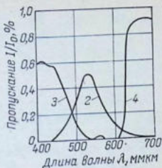
Рис. 4.28. Спектральная характеристика светофильтров прибора ФЭК-М (2, 3, 4 — номера светофильтров).
