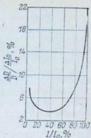
Рис. 4.23. Кривая относительной погрешности в определении оптической плотности.
