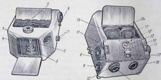
Рис. 4.27. Фотоэлектроколориметр ФЭК-М:
