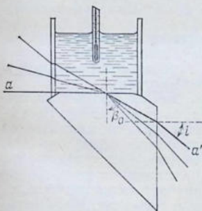
Рис. 3.5. Схема хода лучей в рефрактометре ИРФ-23.
