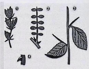
6-rasm. Analogik organlar: 1-zirkning barglari, 2-akastiyaning yonbarglari, 3-do'lana novdasi, 4-atirgul po'stlog'ining tikanlarga aylanishi.
