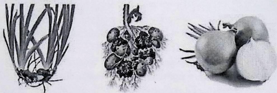
8-Rasm. Poyaning shakl o'zgarishlari: ildizpoya, tuganak, piyozbosh
