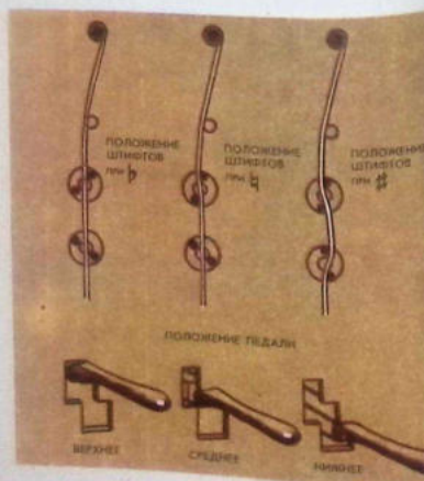
Действие арфового механизма.
