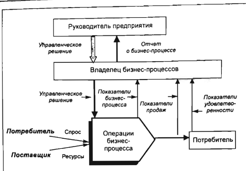
Рис. 2.8. Структура бизнес-процесса
